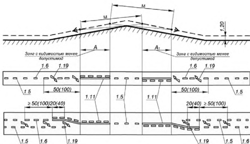
Рисунок А.4 Участки дорог с необеспеченной видимостью
