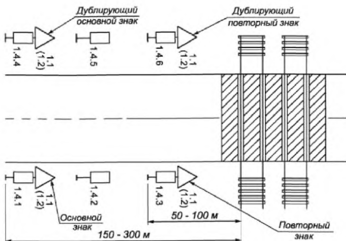
Рисунок А.33 - Размещение знаков 1.4.1-1.4.6
