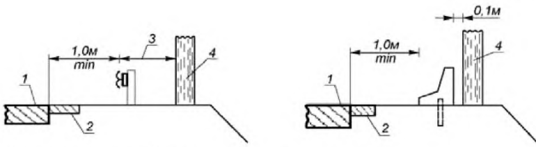
1-проезжая часть; 2-краевая укрепительная полоса; 3-расчетный поперечный прогиб ограждения; 4-препятствие
