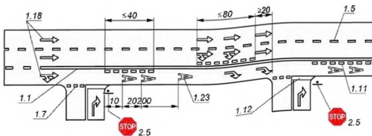
Рисунок А.15 - Маршрутные транспортные средства
