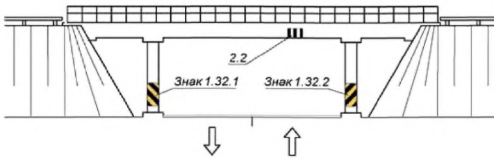
Рисунок А.19 – Объезд препятствия
