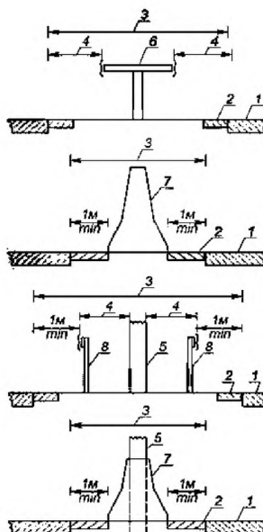
Рисунок А.25 - Расположение светофоров
