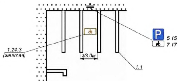
Рисунок А.11 – Знаки «Инвалид»
