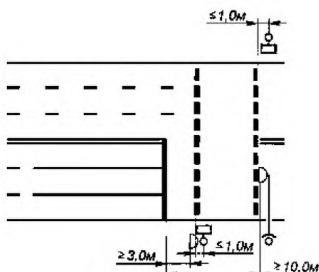
Рисунок А.25 - Расположение светофоров
