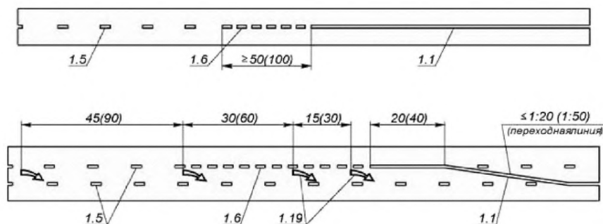
Рисунок А.8 - Перед препятствием
