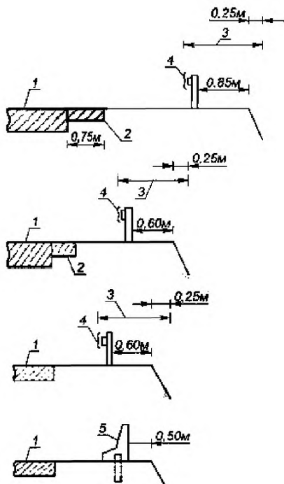
Рисунок А.26 - При наличии опор путепроводов
