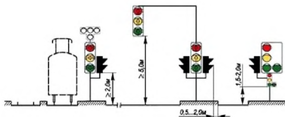
Рисунок А.23 - Самостоятельный светофор
