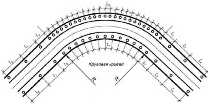
Рисунок А.30 - В пределах кривой в плане и на подходах к ней
