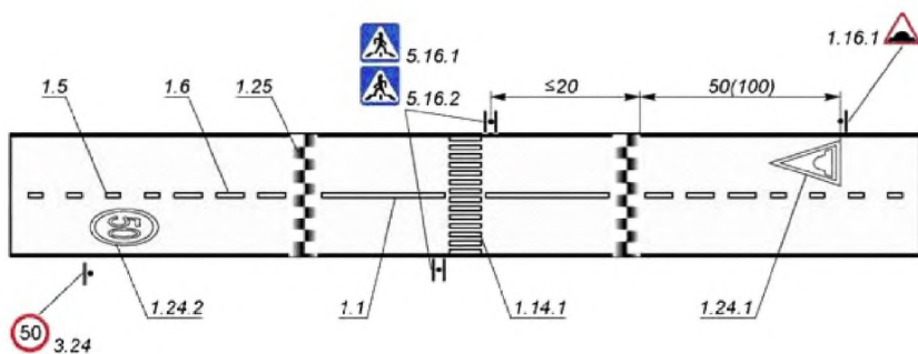
Рисунок А.17 – «Искусственная неровность»
