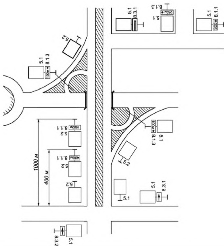
Рисунок А.35 - Пример расстановки знаков 5.1 и 5.2
