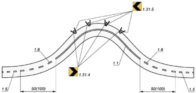
Рисунок А.1 – Направление поворота
