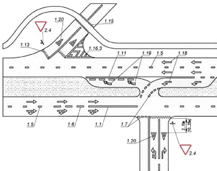
Рисунок А.12 - «Уступите дорогу»
