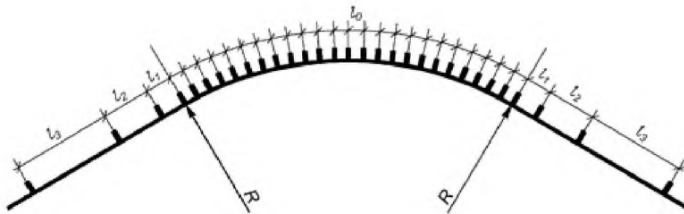
Рисунок А.29 - В пределах кривых в продольном профиле и на подходах к ним
