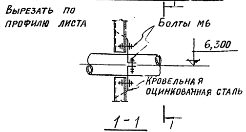
Крайняя цифровая ось ДЕТАЛЬ ЗАДЕЛКИ ОТВЕРСТИЙ В ОБШИВКЕ ДЛЯ ПРОПУСКА ТРУБ
