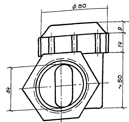
Общий вид
