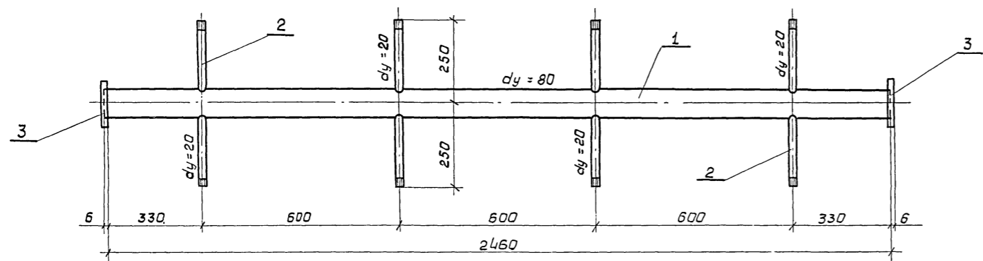
Деталь Т-4
