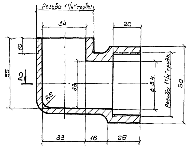
Разрез 1-1
