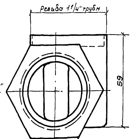
Вид по стр. "А"
