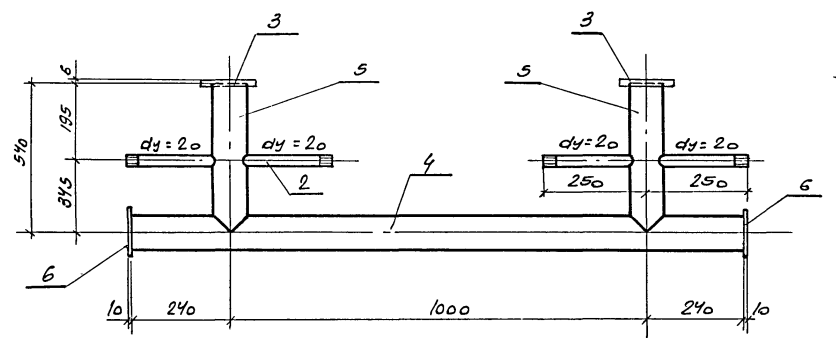
ДЕТАЛЬ Т-2
