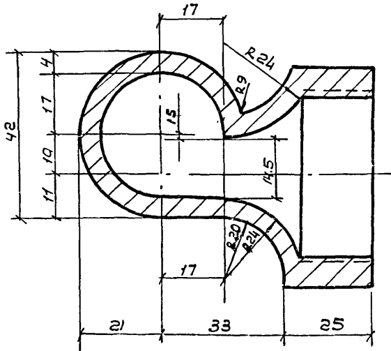
Разрез 2-2
