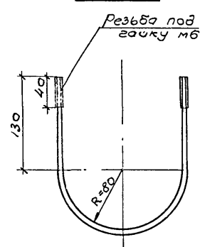
Узел "А" М 1:2
