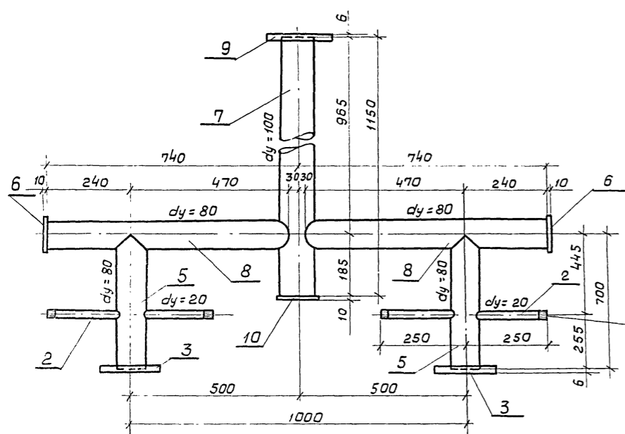
Детали Т-3
