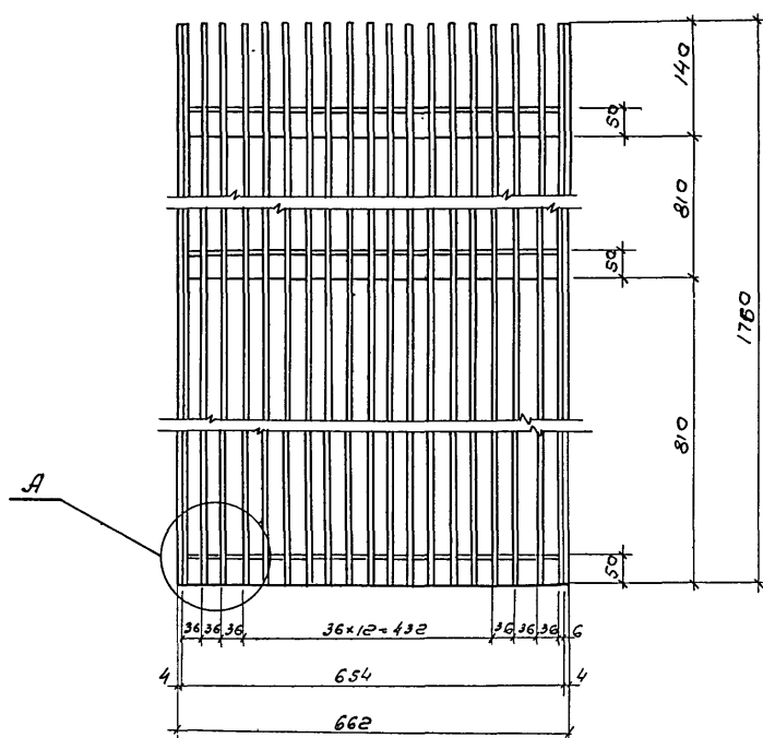
Защитная решетка М 1:10
