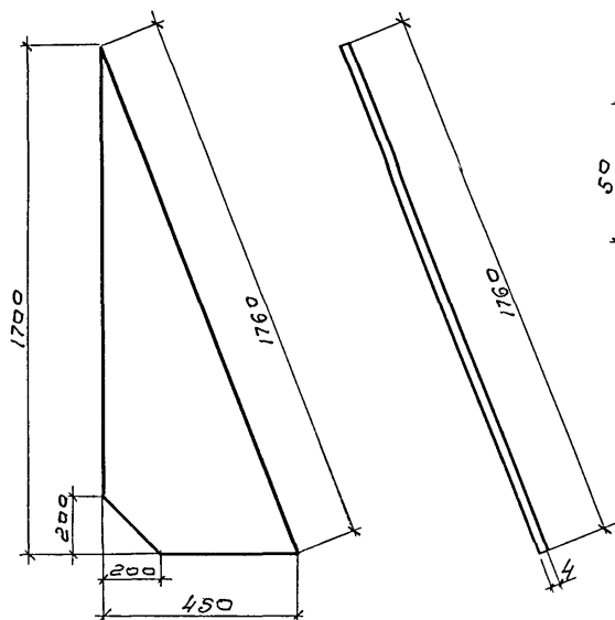
Боковая косынка М 1:20
