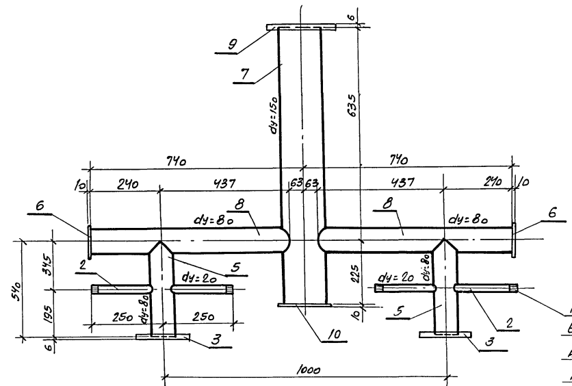
ДЕТАЛЬ Т-3
