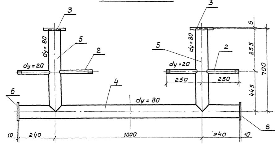
Деталь Т-2
