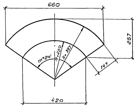
Развертка воронки М 1:10
