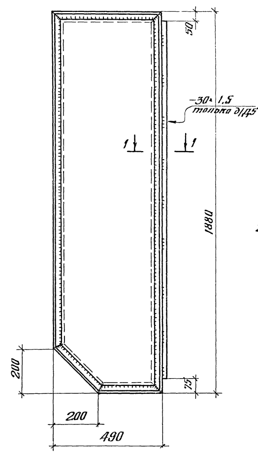
Д5; Д6 (обратна Д5)
