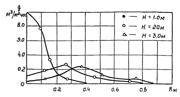
Распределение плотности орошения ρж по радиусу факела разбрызгивания (Rм) при ориентации сопла выходным сечением вниз.
