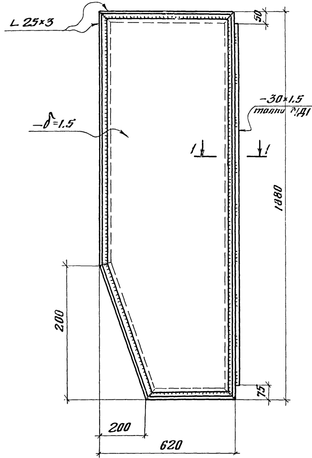
Д1; Д2 (обратна Д1)
