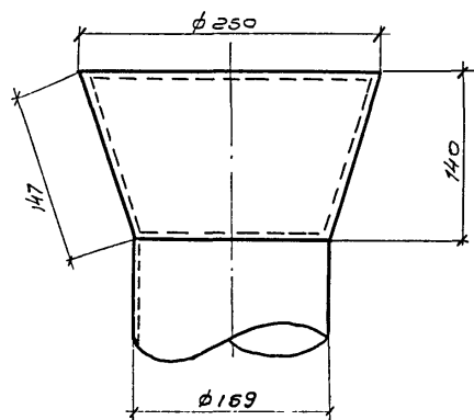
Общий вид воронки М 1:5
