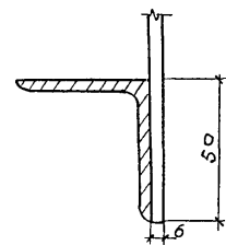
Вид по 3-3
