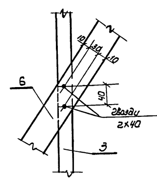
Узел Г М1:10
