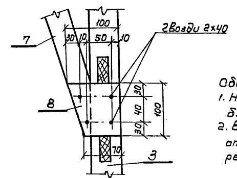
Узел Г М1:10
