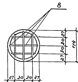
Вид по 2-2 М 1:5
