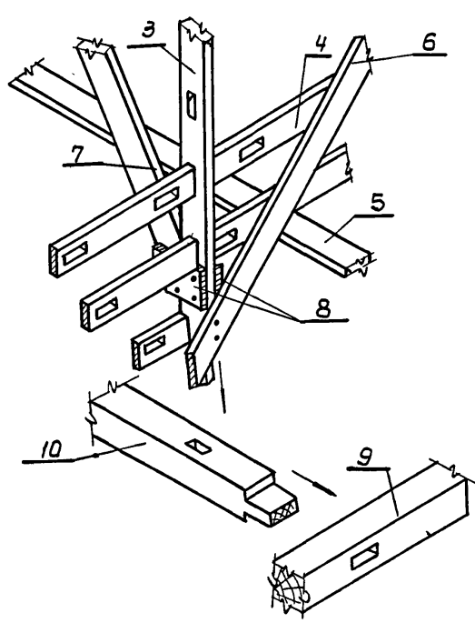
Узел Б М1:10
