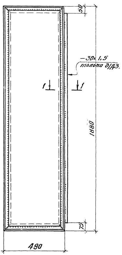
Д3; Д4 (обратна Д3)
