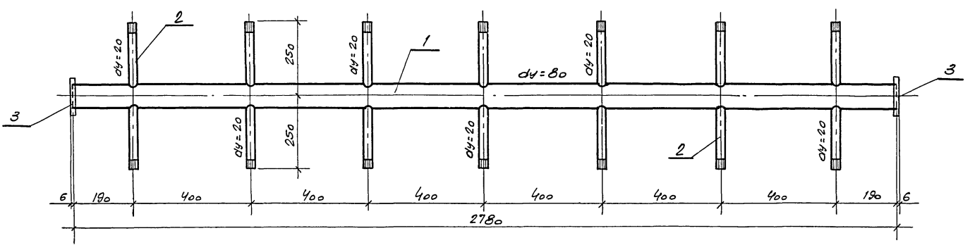
ДЕТАЛЬ Т-2
