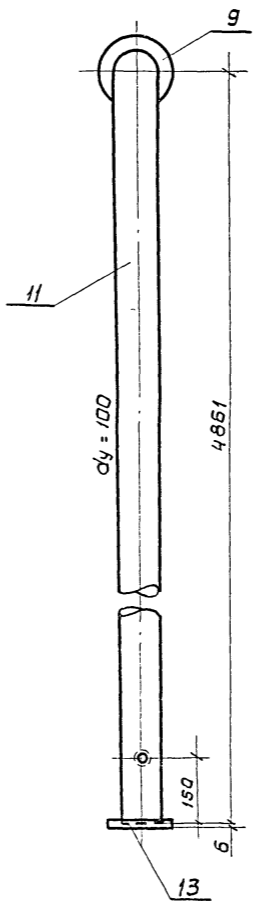
Вид А-А
