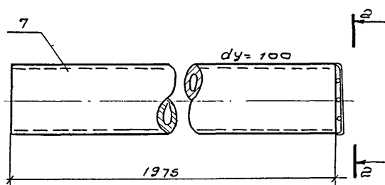
Грязевая труба
