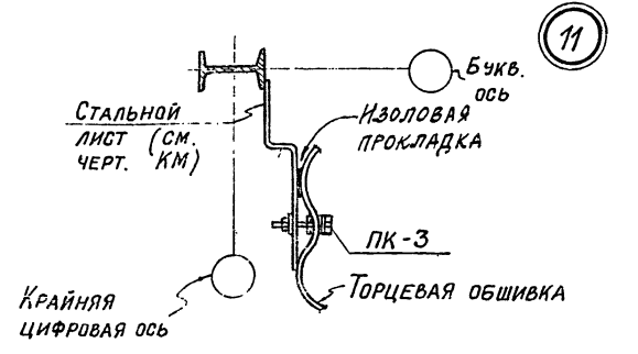
Приборы крепления обшивки см. на листе АС-3.
