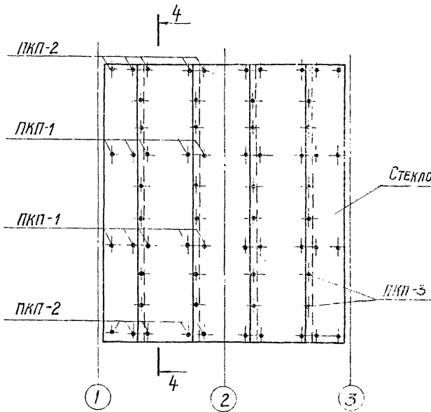
План обшивки их стеклопластика
