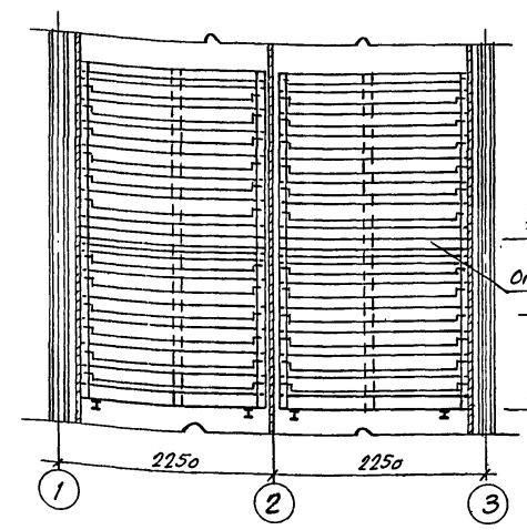
План расстановки щитов пленочного оросителя 2
