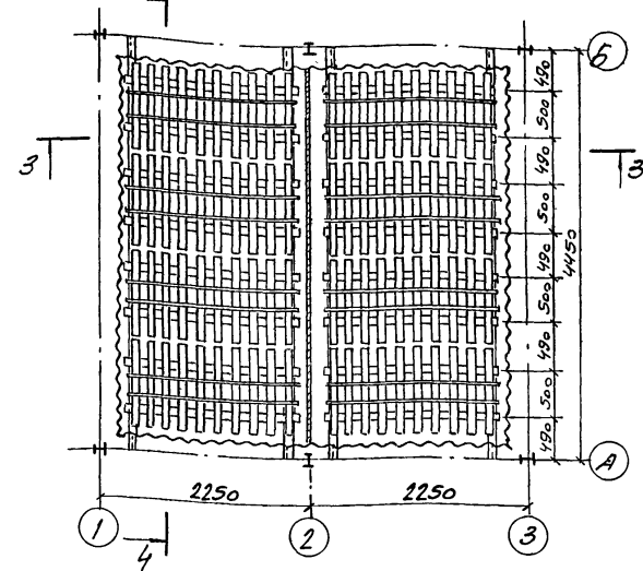
План расстановки блоков капельного оросителя 4
