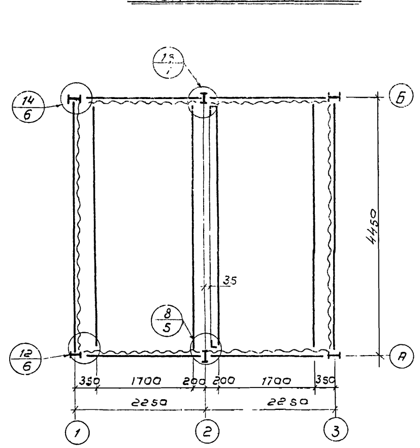
План на отм.+1970
