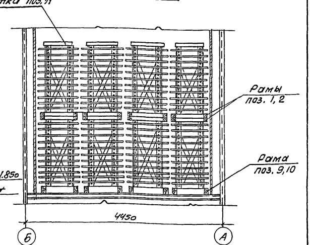
РАЗРЕЗ 4-4
