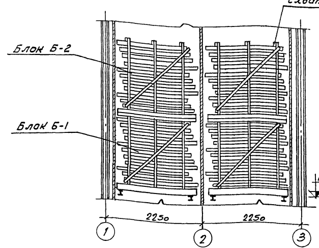
План расстановки блоков капельного оросителя 4
