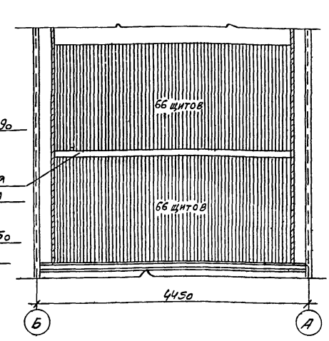
РАЗРЕЗ 2-2
