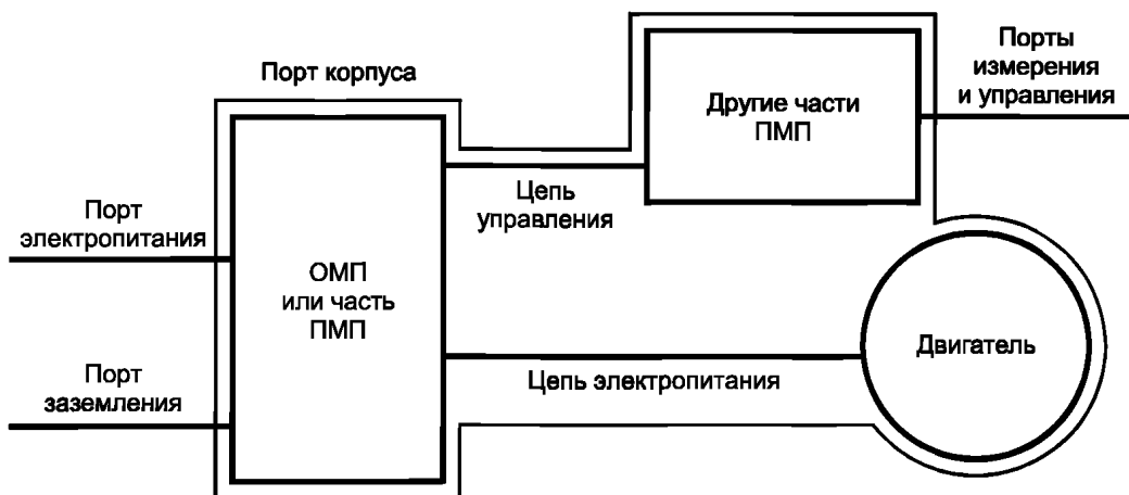
Рисунок 2— Примеры портов СЭП
