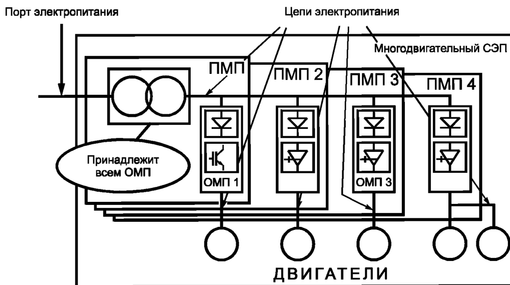
Рисунок 4 — Цепи электропитания СЭП с общим входным трансформатором
