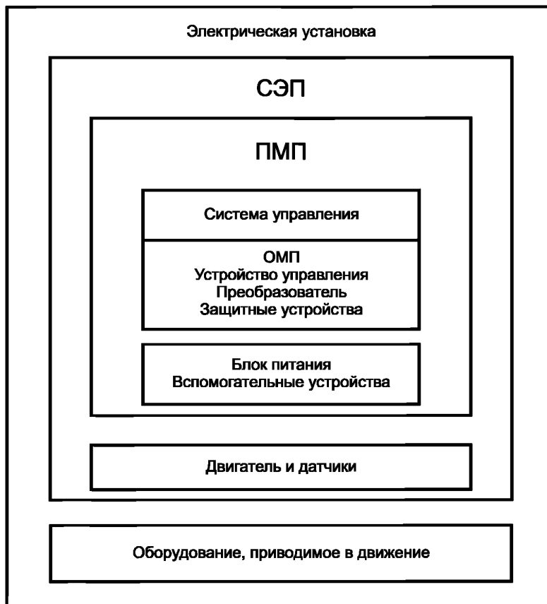
Рисунок 1 — Составные части электрической установки, включающей СЭП
