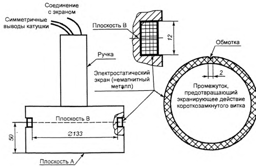
Рисунок А.2 – Конструкция излучающей рамки для неоднородных полей
