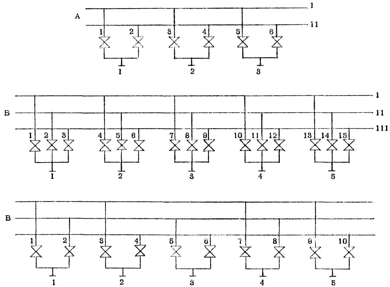
Рис. 7. Традиционные схемы коммутации насосов и трубопроводов.
