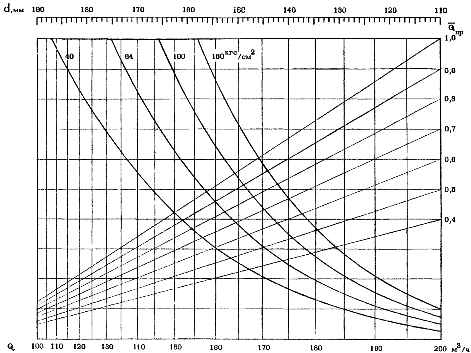
Рис. 3. Номограмма для определения оптимального диаметра трубопровода при подаче насоса 100 - 200 \text{м}^3/\text{ч} .
