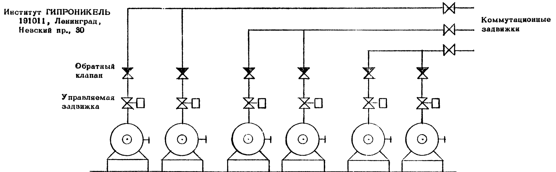
Рис.25. Схема попарного подключения 6-и насосов 14 М 8×4 к 3-м напорным трубопроводам D_y 350 мм
