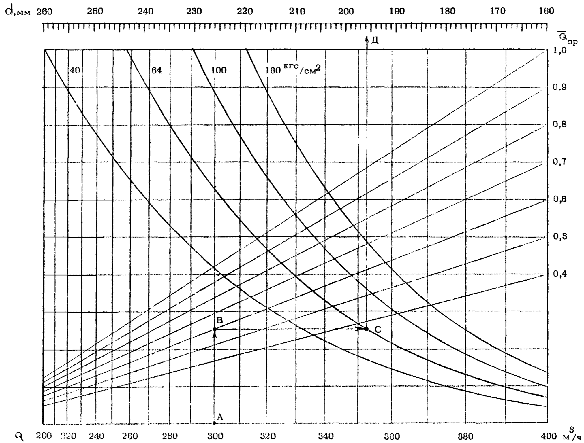
Рис. 4. Номограмма для определения оптимального диаметра трубопровода при подаче насоса 200 - 400 \text{m}^3/\text{ч} .
