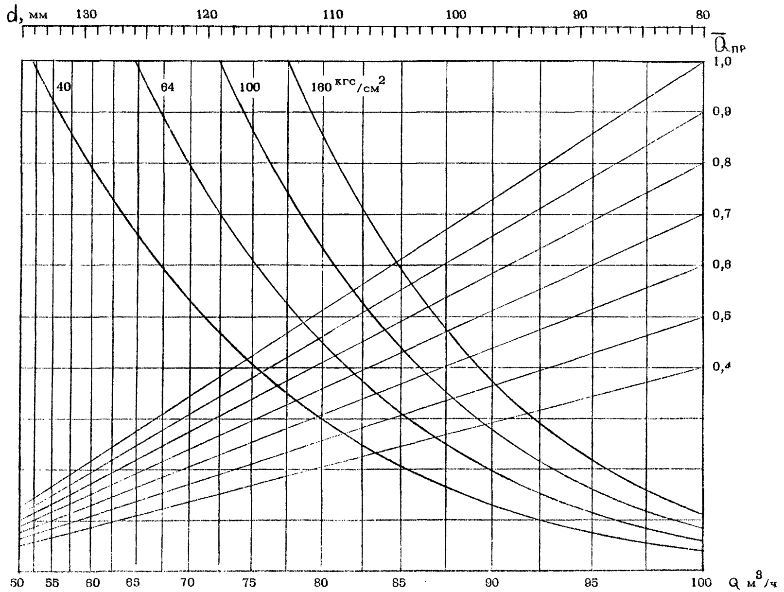
Рис.2. Номограмма для определения оптимального диаметра трубопровода при подаче насоса 50–100 \text{м}^3/\text{ч} .
