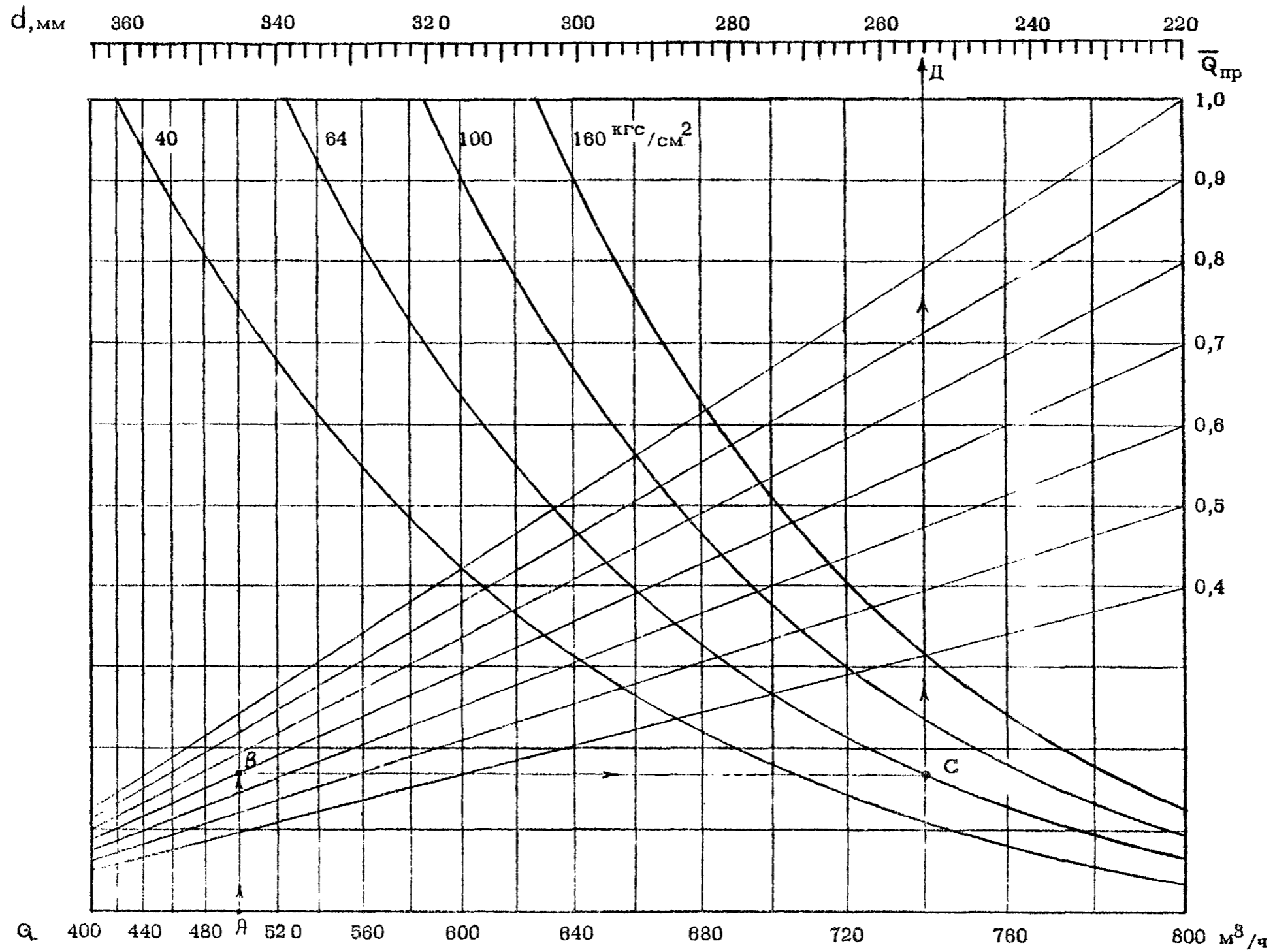
Рис. 5. Номограмма для определения оптимального диаметра трубопровода при подаче насоса 400 – 800 \text{м}^3/\text{ч} .
