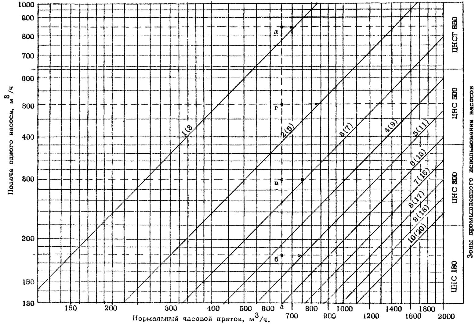
Рис.1. Номограмма для определения числа насосов
