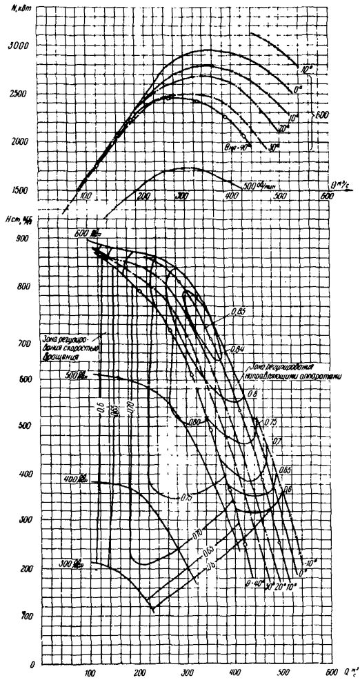
Рис. П. 4. ГЗ. Графики аэродинамических характеристик вентилятора ВЦД-40 при частоте вращения 300–600 об/мин
