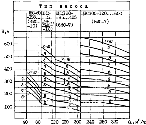
Рис. П.6.1. Напорные характеристики и рабочие зоны насосов:
