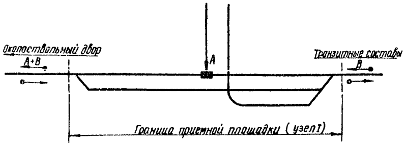
Рис.2. Схема приемной площадки, расположенной на основной транспортной магистрали
