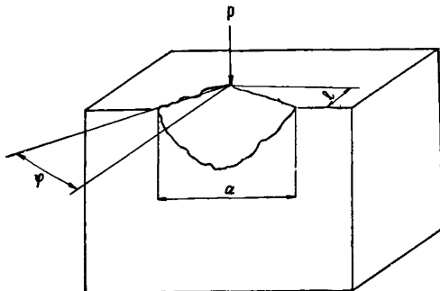
Схема испытания горных пород на статическое откалывание
