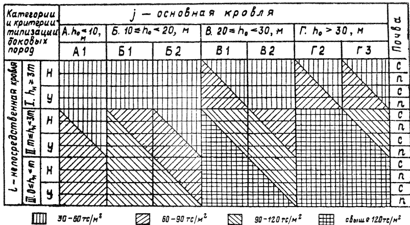
Рис. 5.2. Распределение прогнозируемых уровней сопротивления механизированной крепи по типам кровли
