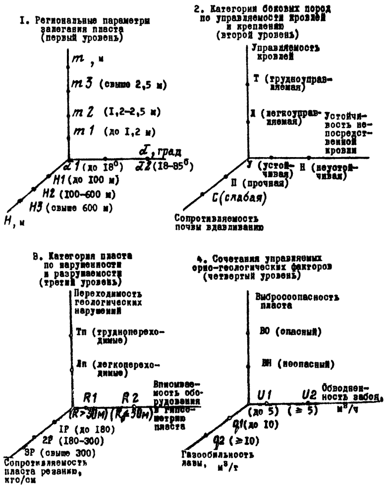
Рис. 3.1. Классификация горно-геологических условий эксплуатации механизированных комплексов
