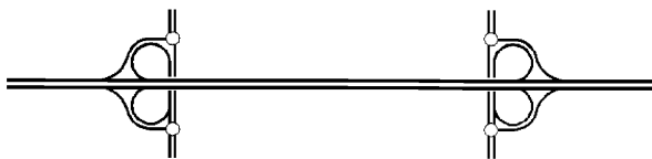
Рисунок 10.2 – Схема транспортных развязок «Разделенный неполный клеверный лист»
