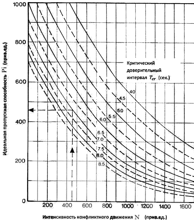
Рисунок Ю.7 – Диаграмма для определения идеальной пропускной способности движения на пересечении
