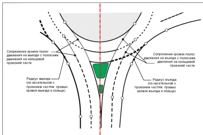
Рисунок К.13 – Схема сопряжения кромок полос движения участка въезда-въезда с кромками полос движения кольцевой проезжей части двухполосного кольцевого пересечения
