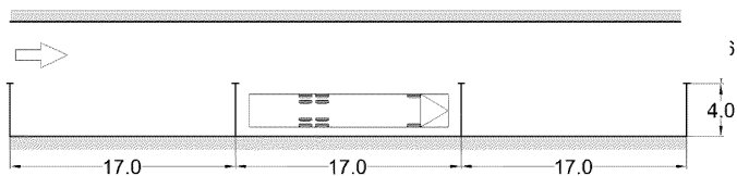
Рисунок Б.5 – Размеры парковочных мест при продольном размещении автобусов (А)
