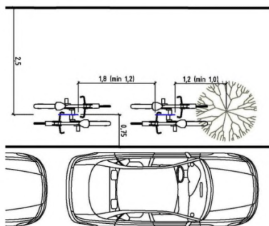
Рисунок Л.26 – Пример расположения велостоянок параллельно проезжей части
