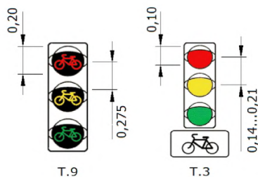
Рисунок Л.17 – Габариты светофоров Т.9 и Т.3 с табличкой 8.4.7 (ПДД)
