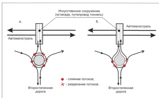
Рисунок 9.19 – Конфликтные точки на примыкании съездов к второстепенной улице или дороги неполных транспортных развязок при центральном островке круглой (а) и каплеобразной (б) формы
