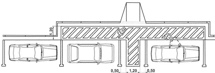
Рисунок Ы.14 – Схема планировки парковочных мест параллельно тротуару на левой стороне проезжей части улицы с односторонним движением, оборудованной «карманом» для подхода инвалидов к транспортным средствам
