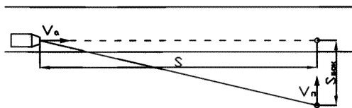
Рисунок 7.13 – Схема для определения минимального расстояния боковой видимости у пешеходного перехода
