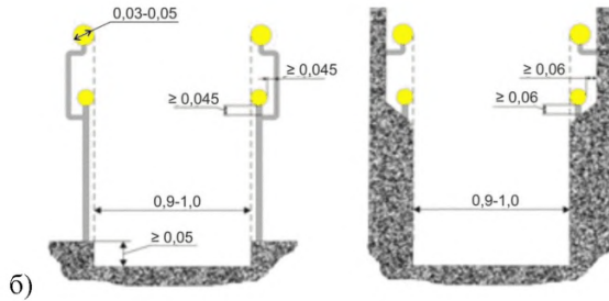
Рисунок 14.3 – Параметры поручней
