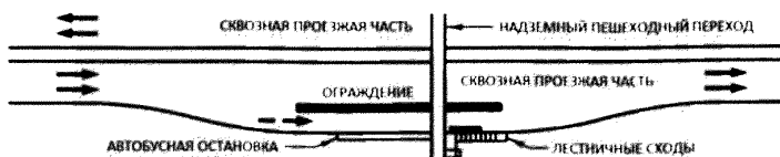
Рисунок 11.4 – Остановочный пункт на обособленном проезде
