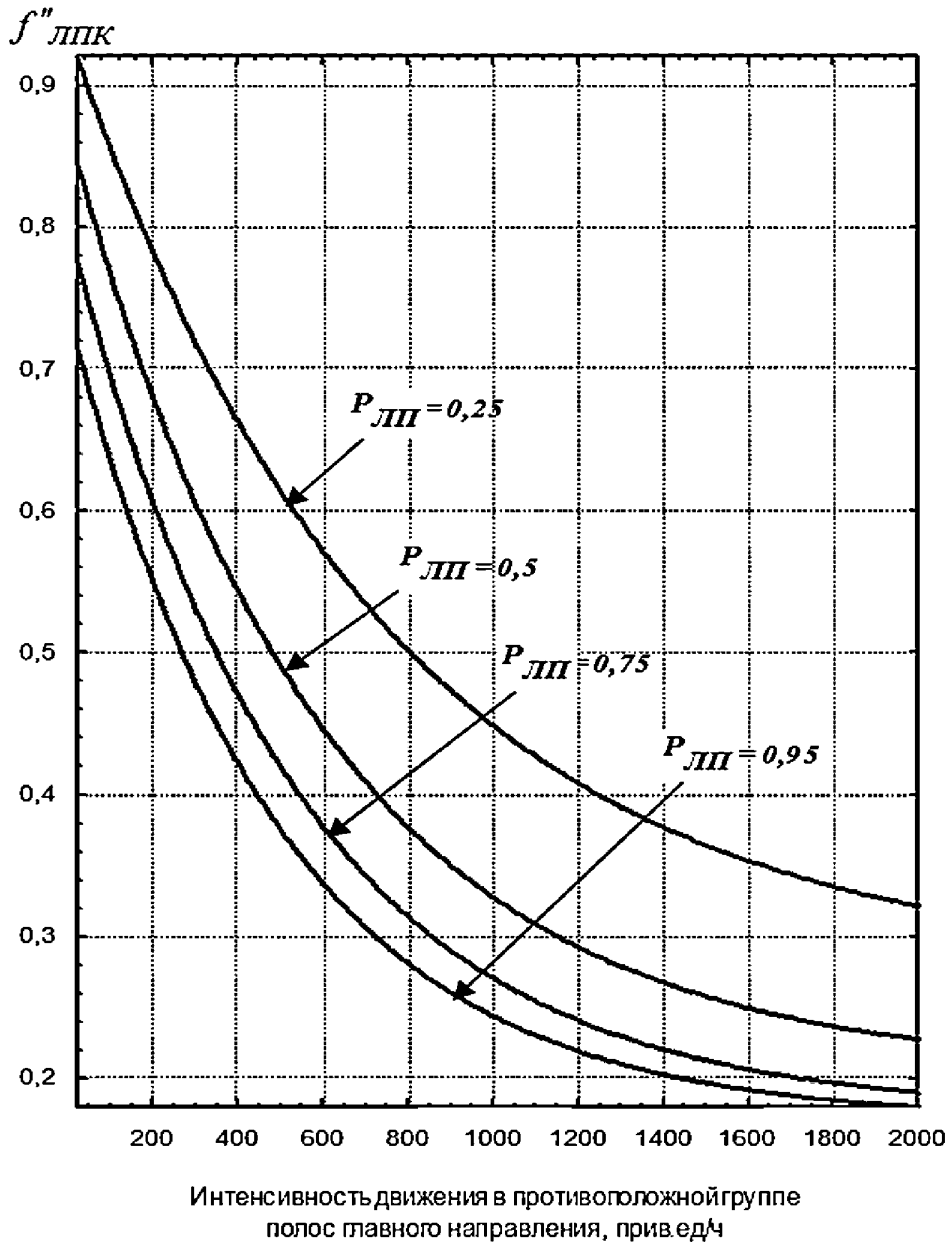
Рисунок Г.4 – Графики зависимости коэффициента f''_{ЛПК} от интенсивности противоположного потока N_{пр} , соотношение количества полос движения n = 1 , n_{пр} = 1
