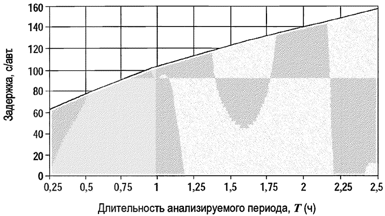
Рисунок Г.21 – Чувствительность задержки к длине анализируемого периода
