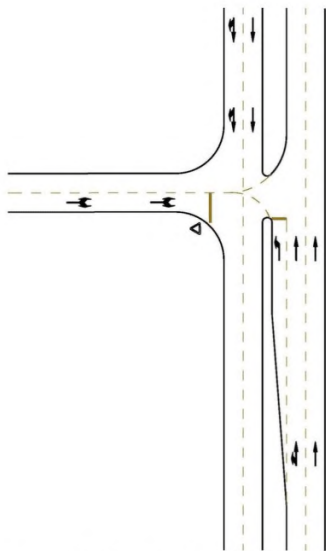
Рисунок Ю.11 – Применение специальной полосы для поворота налево на улице с разделенными проезжими частями и шириной разделительной полосы не менее 5,0 м
