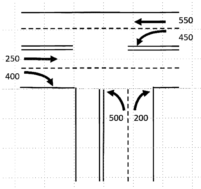
Рисунок Ю.10 – Данные для примера расчета светофора
