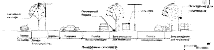
Рисунок Р.13 – Примеры планировочных решений зон посадки и высадки пассажиров такси, личных автомобилей
