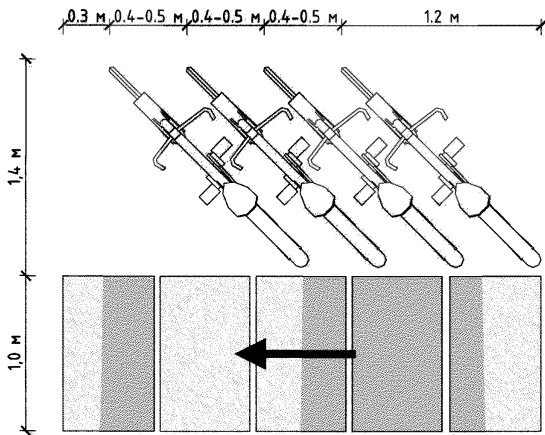
Рисунок Л.24 – Парковочное пространство при диагональном расположении велосипедов
