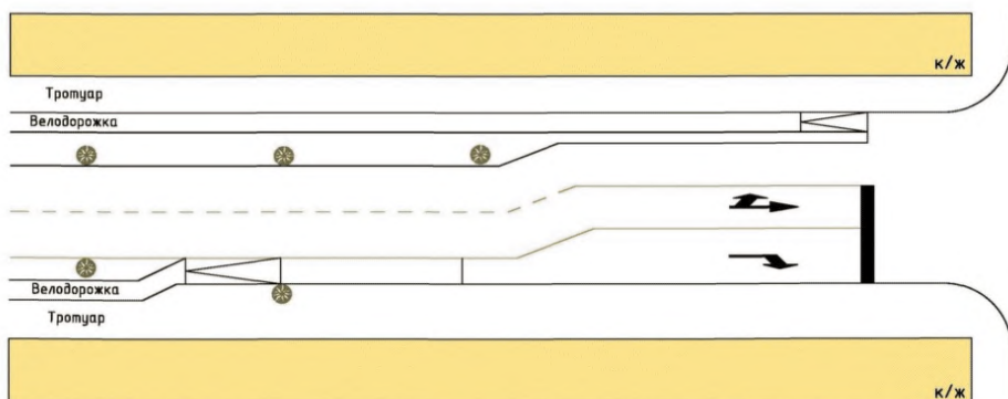
Рисунок Л.7 – Пример расширения проезжей части с устройством полосы для правых поворотов
