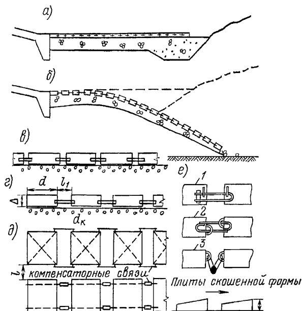
Рисунок 4.24 – Конструкция переходного крепления из каменной наброски, покрытой бетонными плитами с компенсационными связями: а – продольный разрез до начала размыва; б – то же после размыва русла и деформации крепления; в – вид плит с компенсаторными связями до раздвижки; г – то же после раздвижки; д – план фрагментов с боковыми и торцевыми компенсаторными связями; е – варианты конструкций компенсаторных связей; 1 – по бокам плит; 2 – по верху плит; 3 – между плитами
