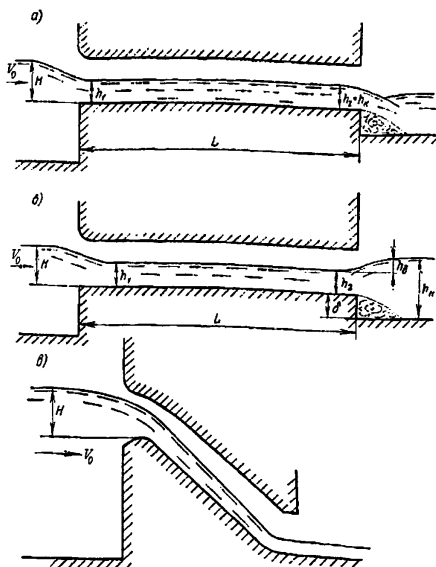
Рисунок 3.4 – Истечение через трубчатый водосброс по схеме водослива:
