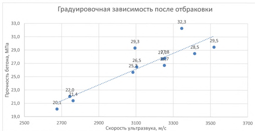
Рисунок 3.14 – График градуировочной зависимости после отбраковки
