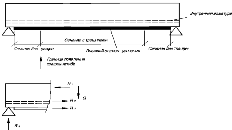
Рисунок 25 – Разделение анкеровки на границе возникновения трещин:
