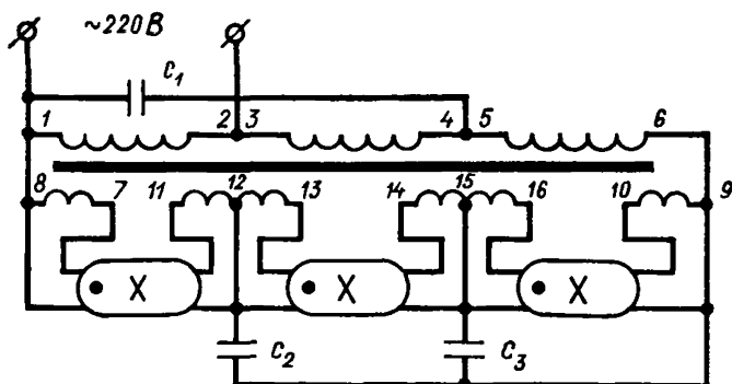
Рис. 3. Принципиальная схема включения люминесцентных ламп с пускорегулирующим аппаратом в виде автотрансформатора с повышенным рассеянием
