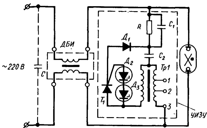
Рис. 2. Принципиальная схема включения ламп ДНаТ и ДРИ с импульсным зажиганием
