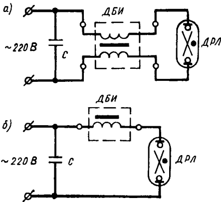
Рис. 1. Принципиальная схема включения ламп ДРЛ без повышенного напряжения зажигания а — дроссель с симметричными обмотками; б — дроссель с несимметричными обмотками
