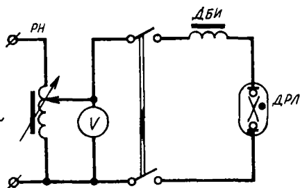
Электрическая схема контроля напряжения зажигания ламп ДРЛ
