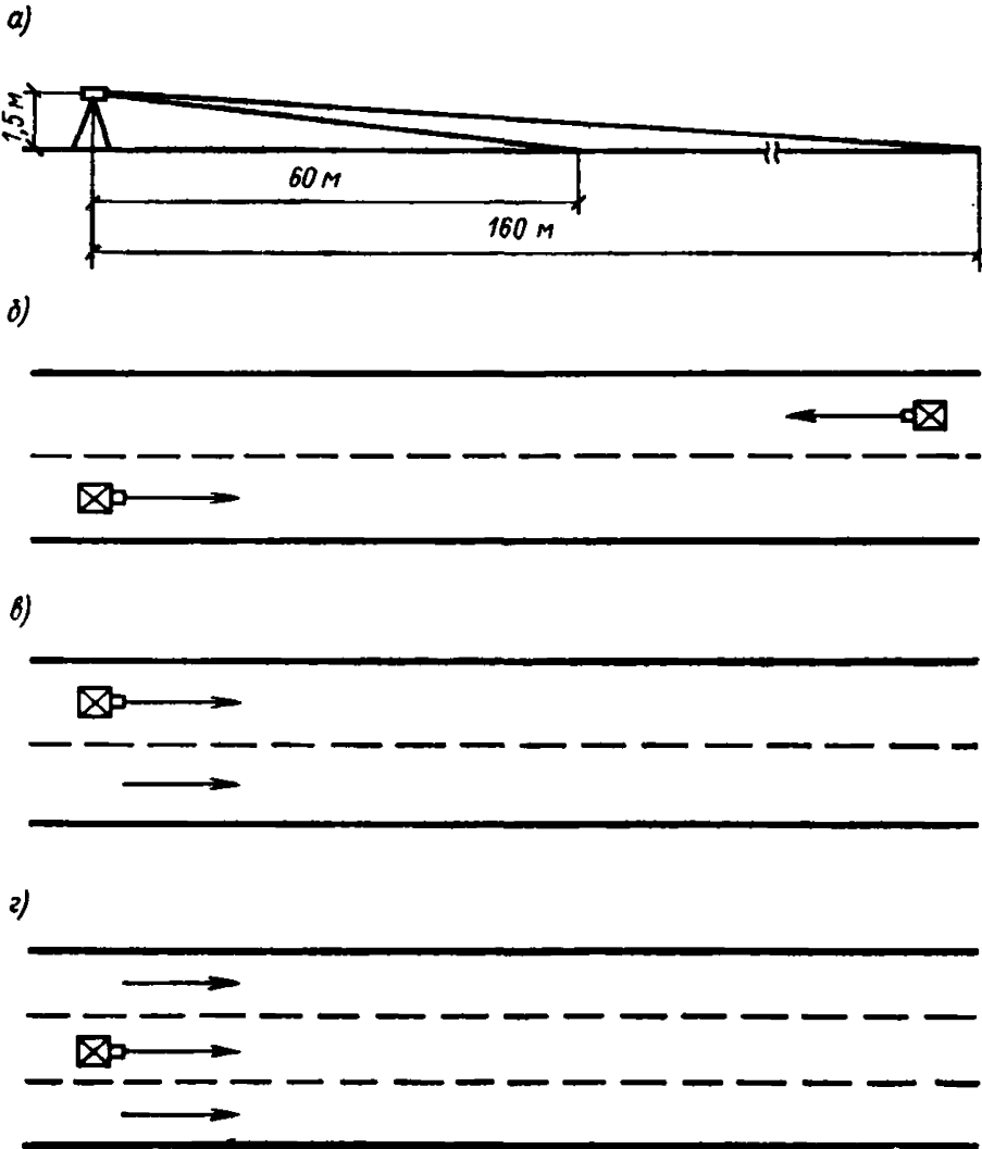
Рис. 2. Положение яркомера при измерении яркости покрытий дороги в зависимости от числа полос и направлений движения
