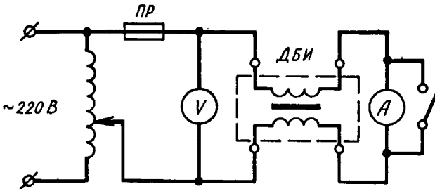
Принципиальная схема измерения контрольных точек дросселя
