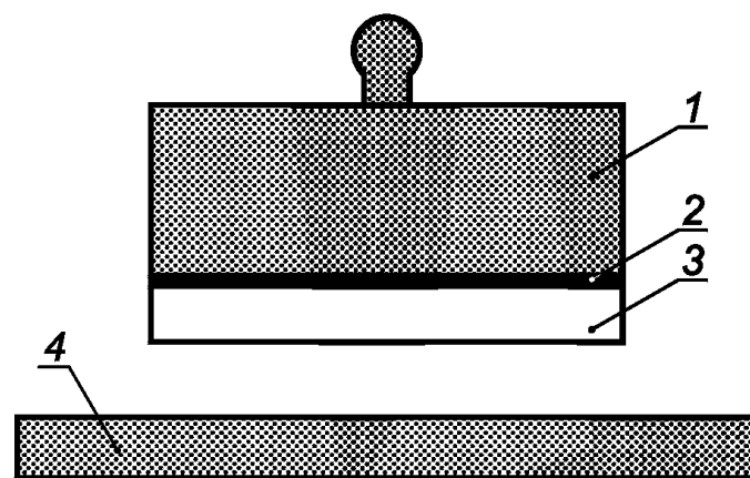
а) АТС-1 — отрыв по границе «образец — основание»
