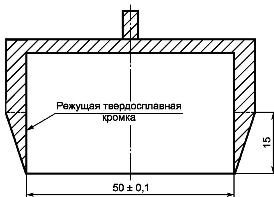
Рисунок 2 — Сверло-коронка с режущей твердосплавной кромкой
