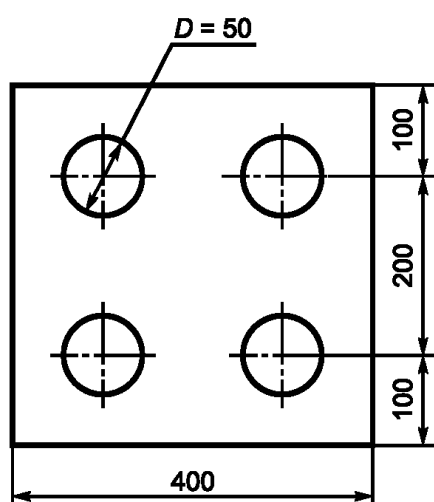
Рисунок 3 — Расположение анкеров на поверхности образца
