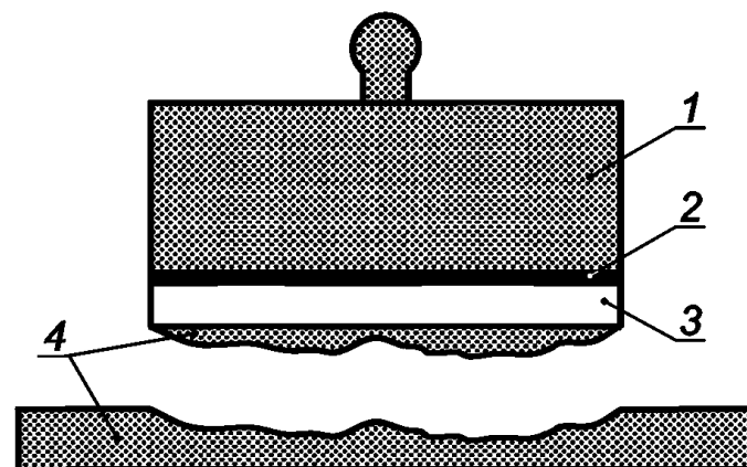
в) АТС-3 — отрыв по телу основания
