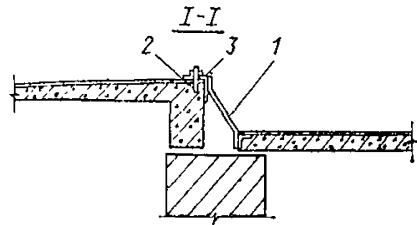
РИС. 4. УСТРОЙСТВА ДЛЯ ВРЕ- МЕННОГО КРЕПЛЕНИЯ КАРНИЗ- НОГО БЛОКА
