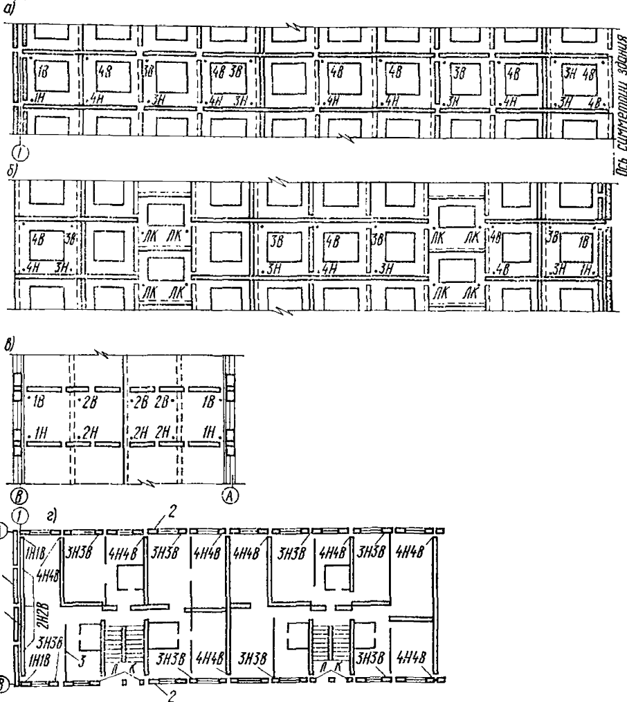
РИС. 1. РАСПОЛОЖЕНИЕ СТАЛЬНЫХ ЭЛЕМЕНТОВ В НАРУЖНЫХ СТЕНАХ
