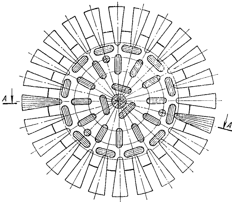
РИС. 4. ЩЕТКА
