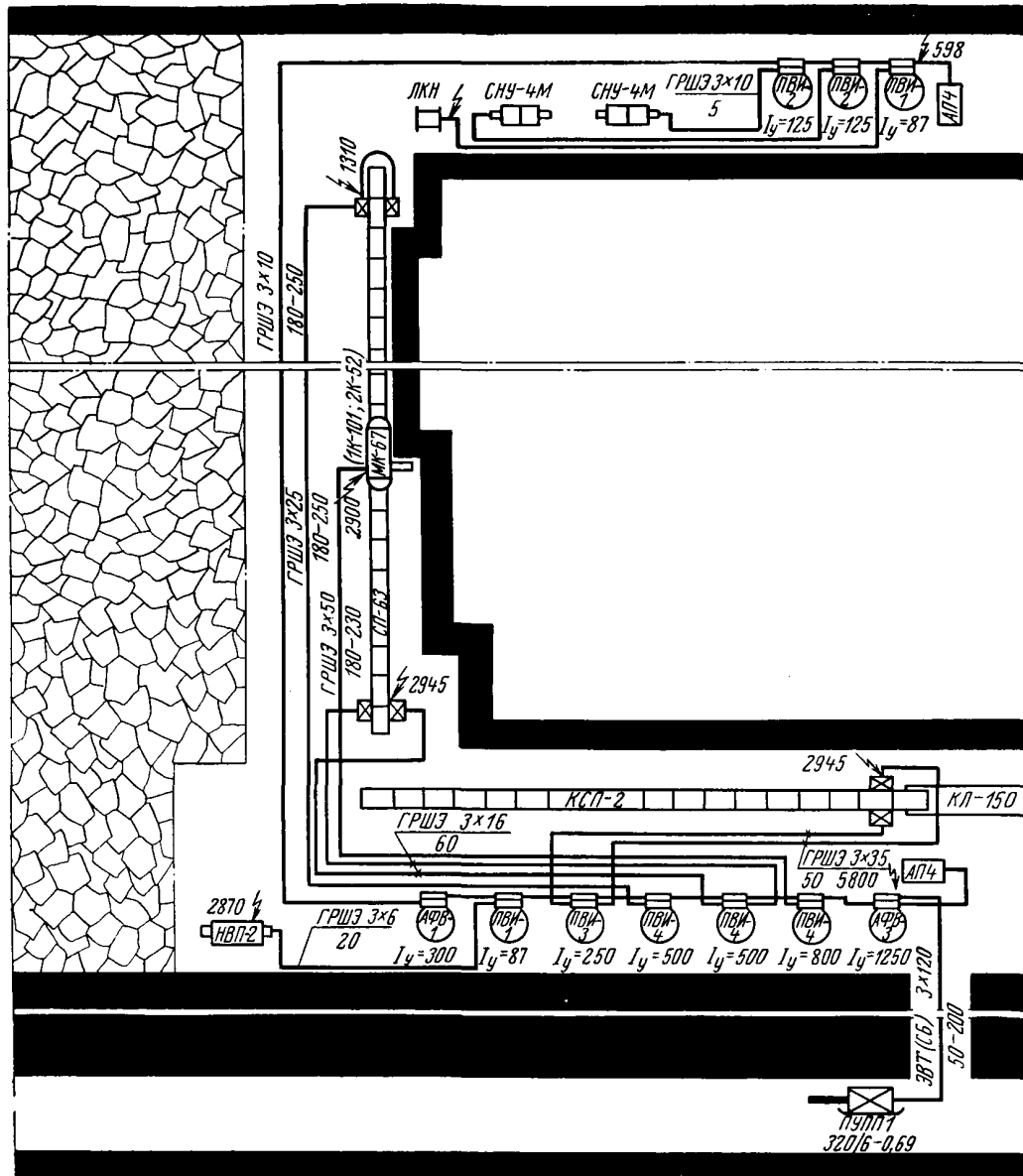
Схема электроснабжения очистного забоя
