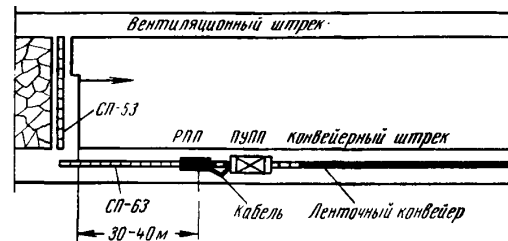
Рис. 2. Установка ПУПП над скребковым конвейером
