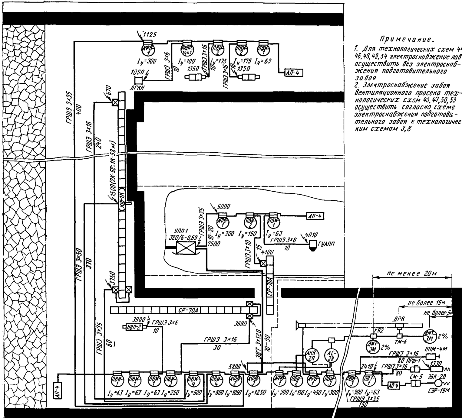
Схема электроснабжения очистного участка
