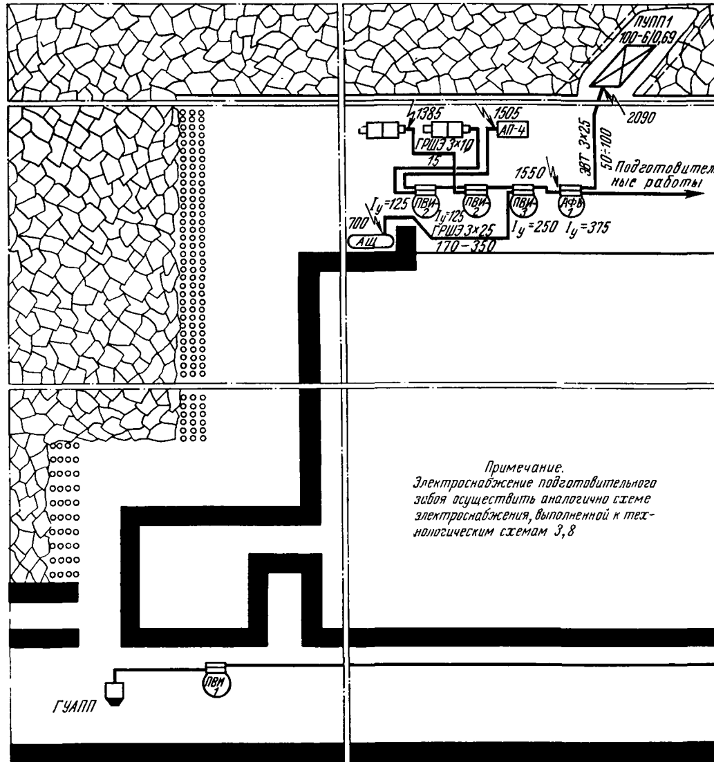
Схема электроснабжения очистного зобоя
