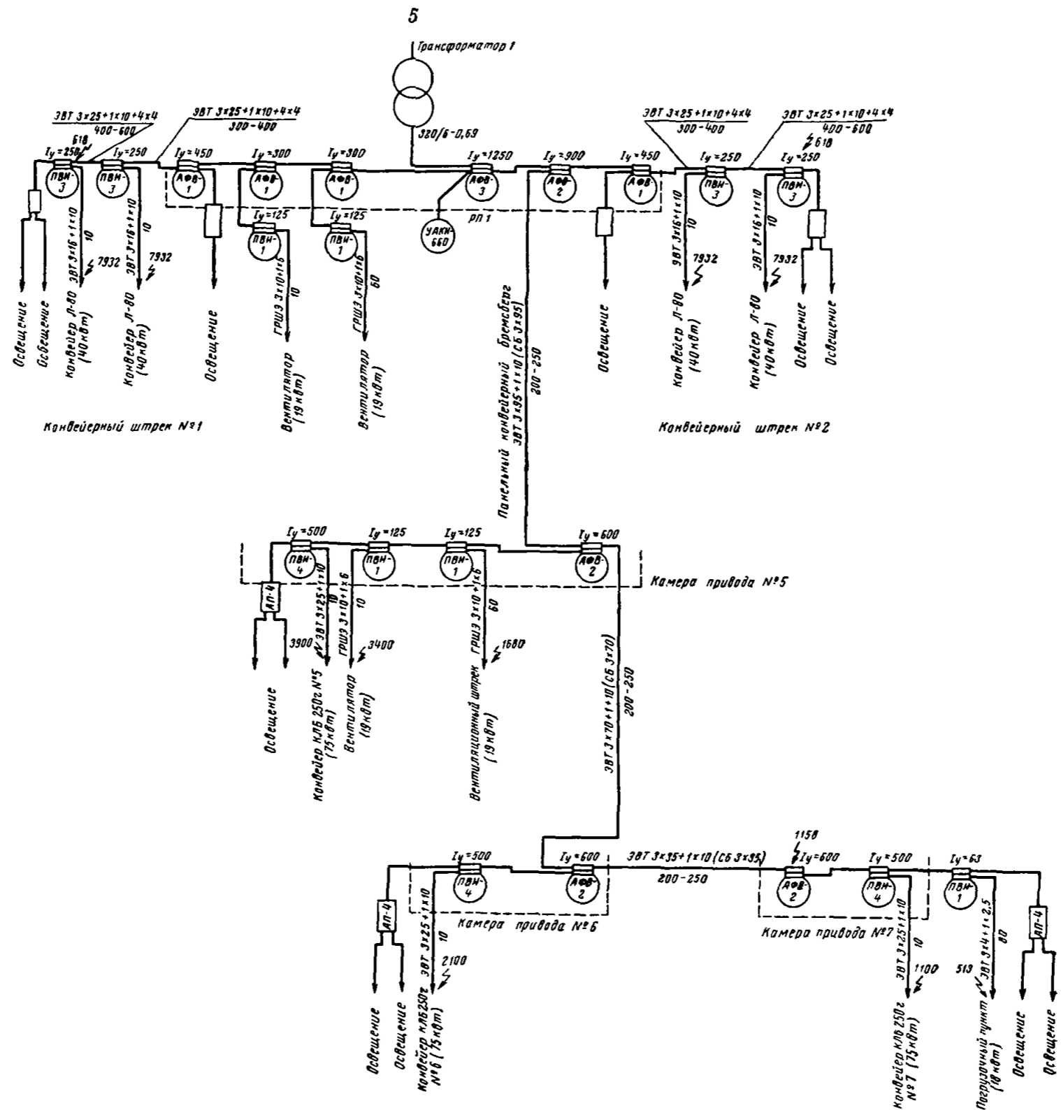
Общая принципиальная схема электроснабжения тормозного поля для технологических схем № 1, 2, 7, 29
