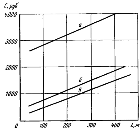
Рис. 1. Годовые затраты при раздельной и совмещенной установках (над конвейером) ПУПП и РПП-0,66 кв при различных расстояниях между ними:
