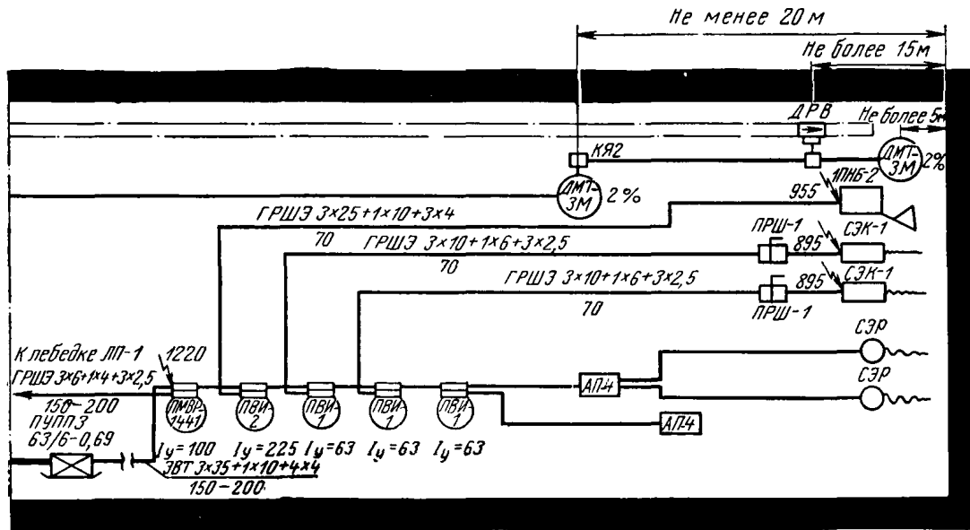
Схема электроснабжения подготовительного забоя
