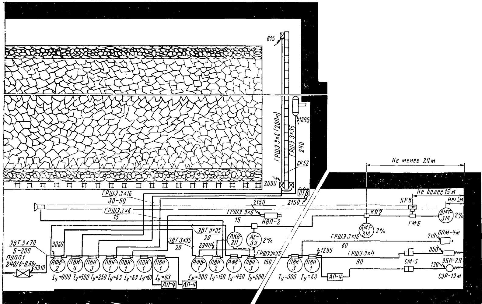
Схема электроснабжения участка
