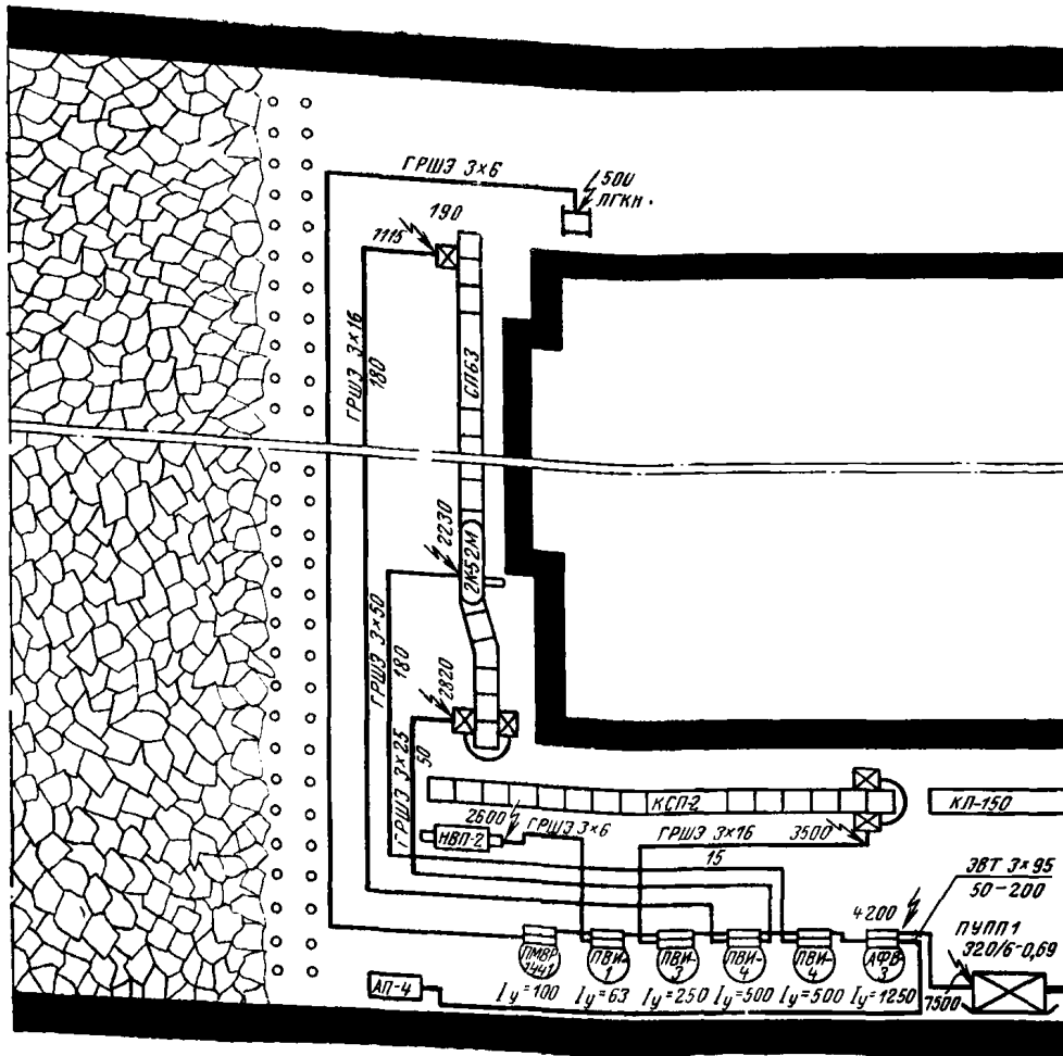
Схема электроснабжения очистного забоя верхнего слоя
