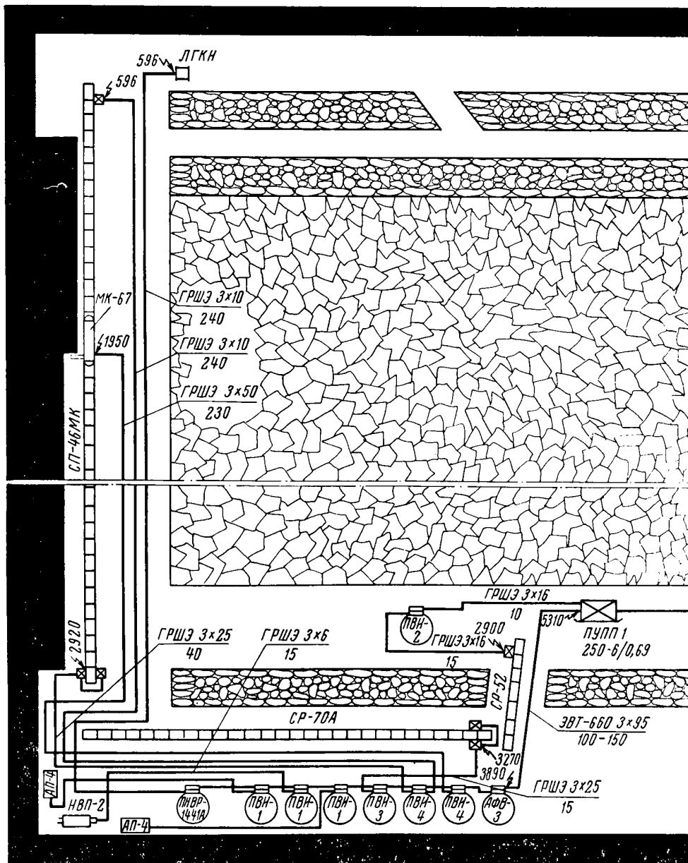
Схема электроснабжения очистного участка
