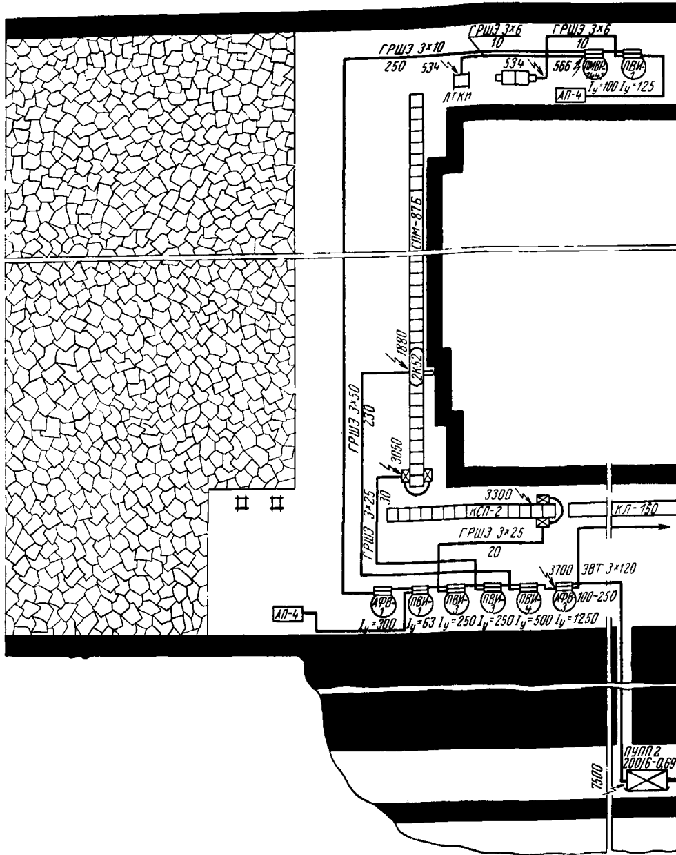
Схема электроснабжения очистного забоя
