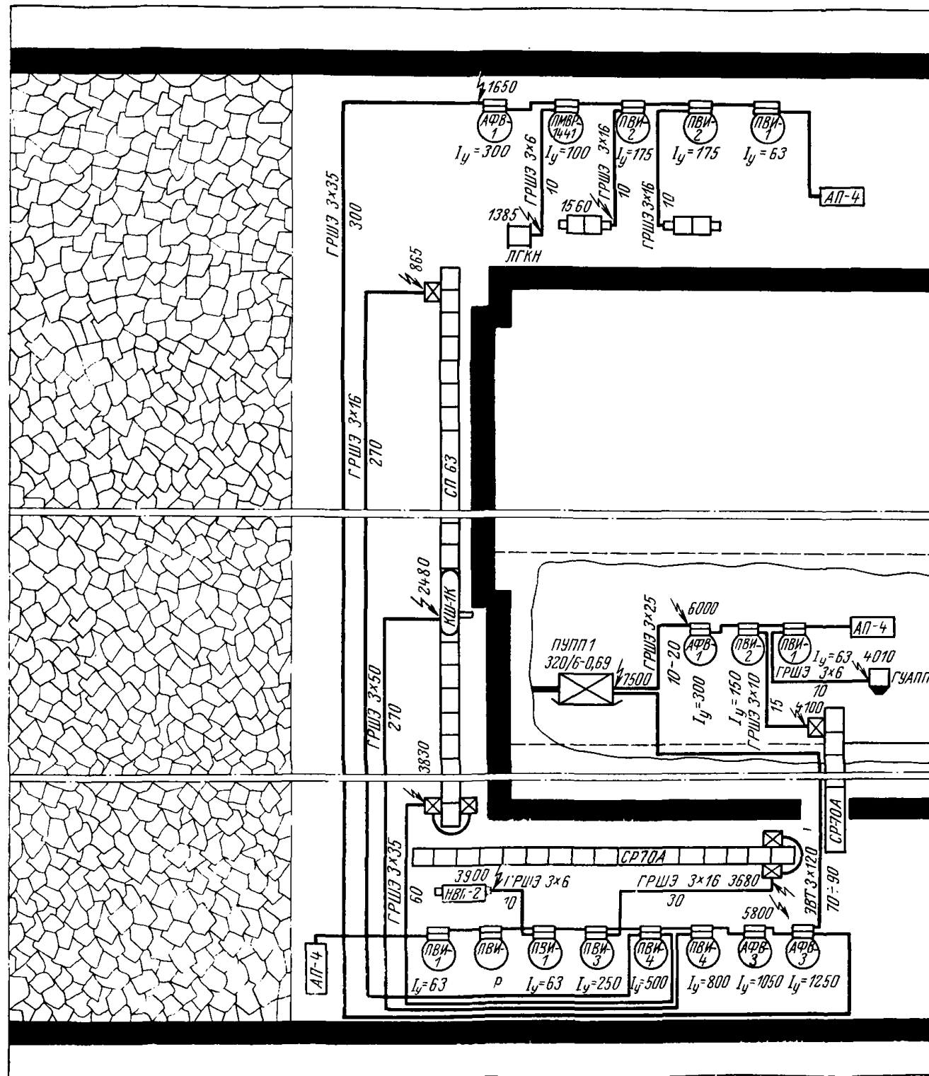
Схема электроснабжения очистного забоя
