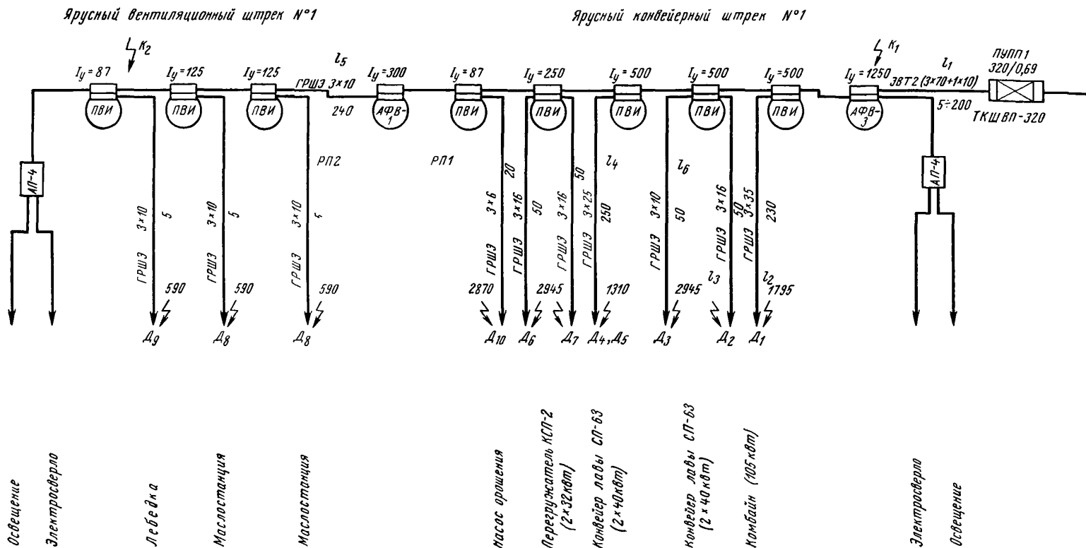
Рис. 4. К расчету системы электроснабжения участка угольной шахты
