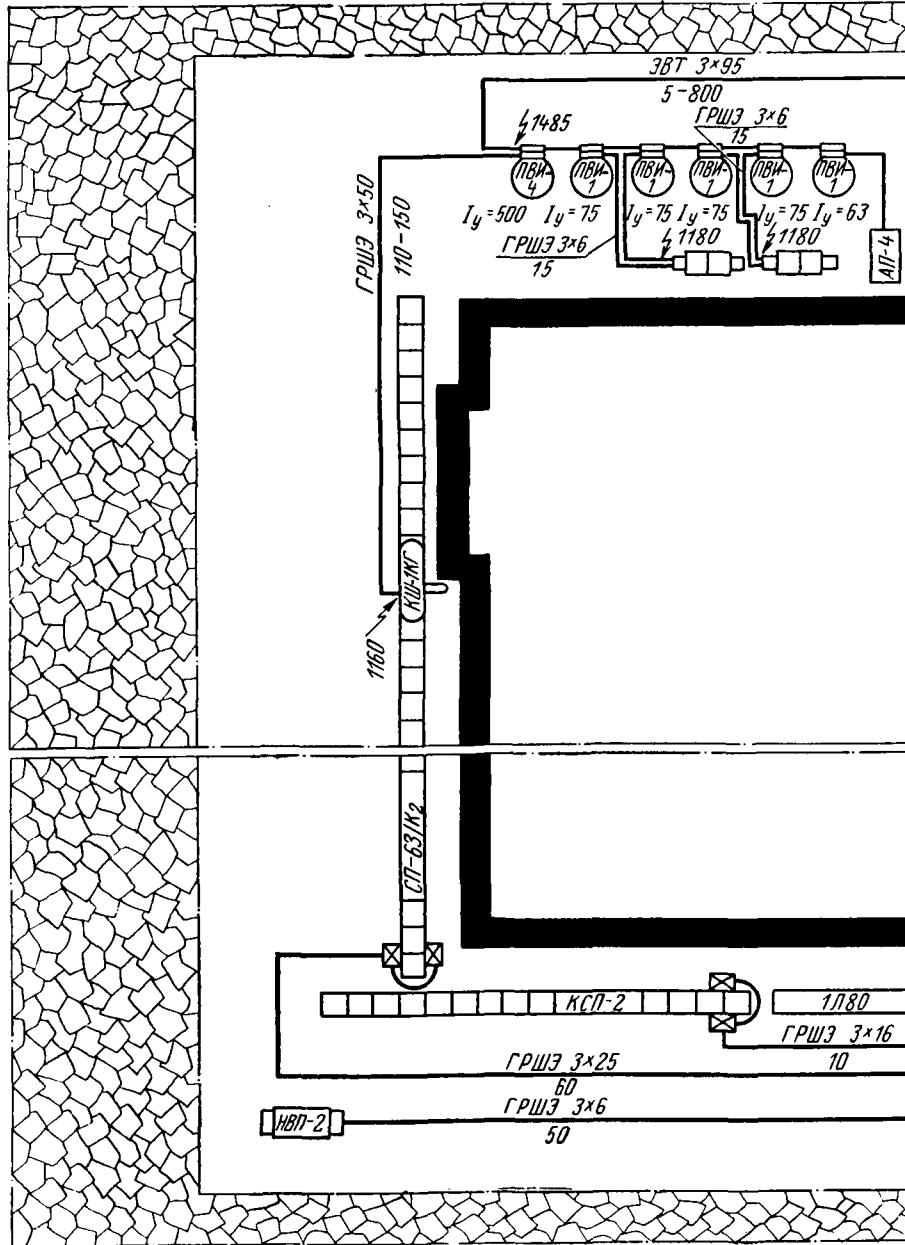
Схема электроснабжения очистного забоя
