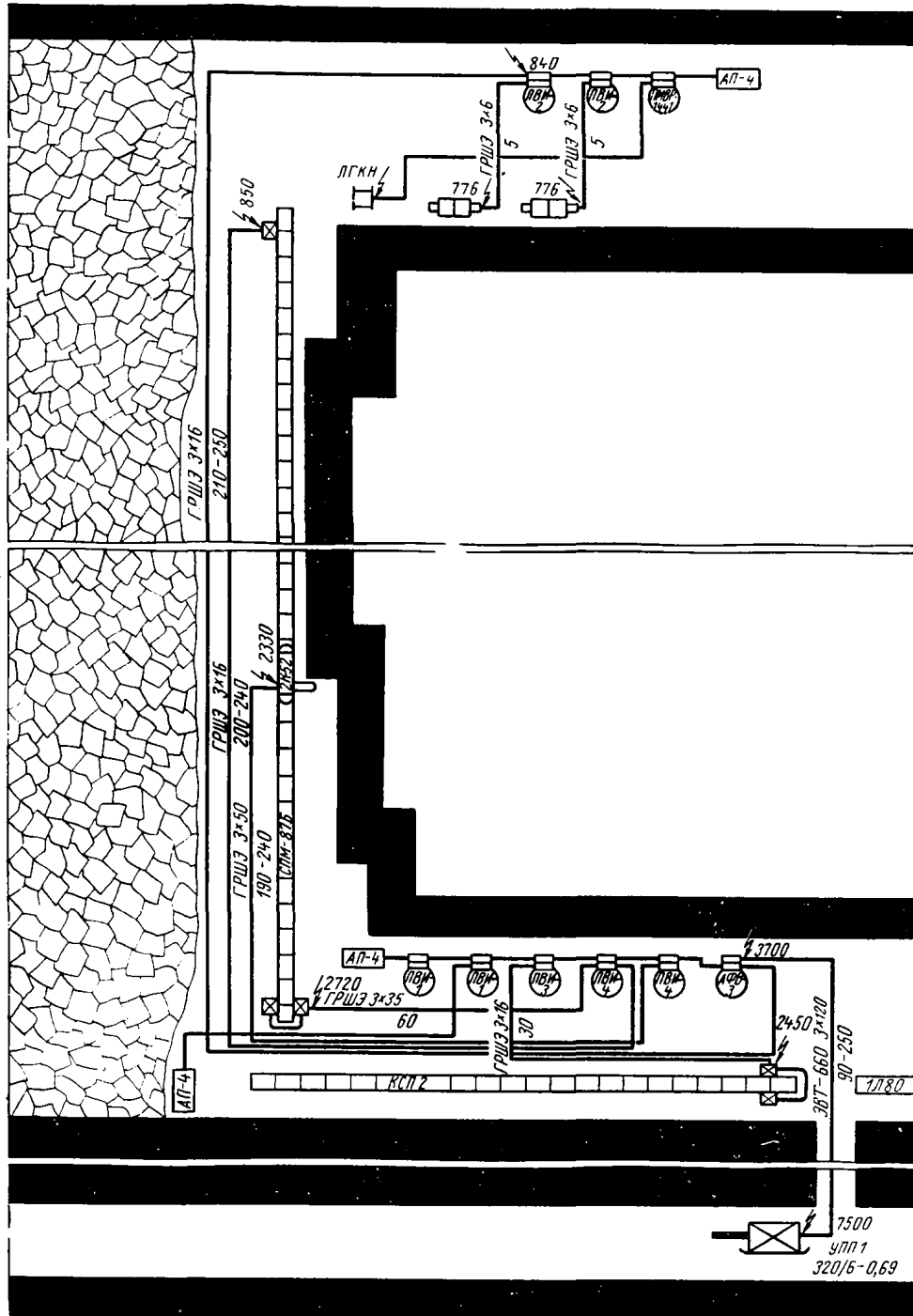
Схема электроснабжения очистного забоя
