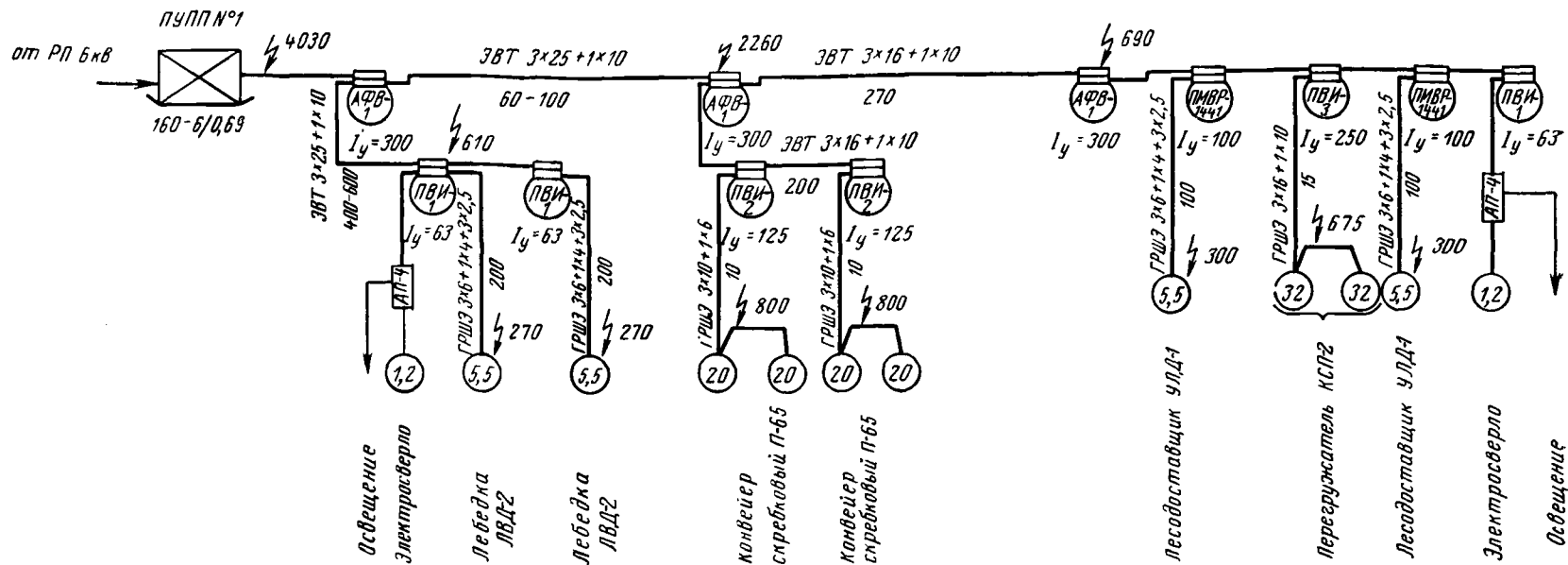
Принципиальная схема электроснабжения участка
