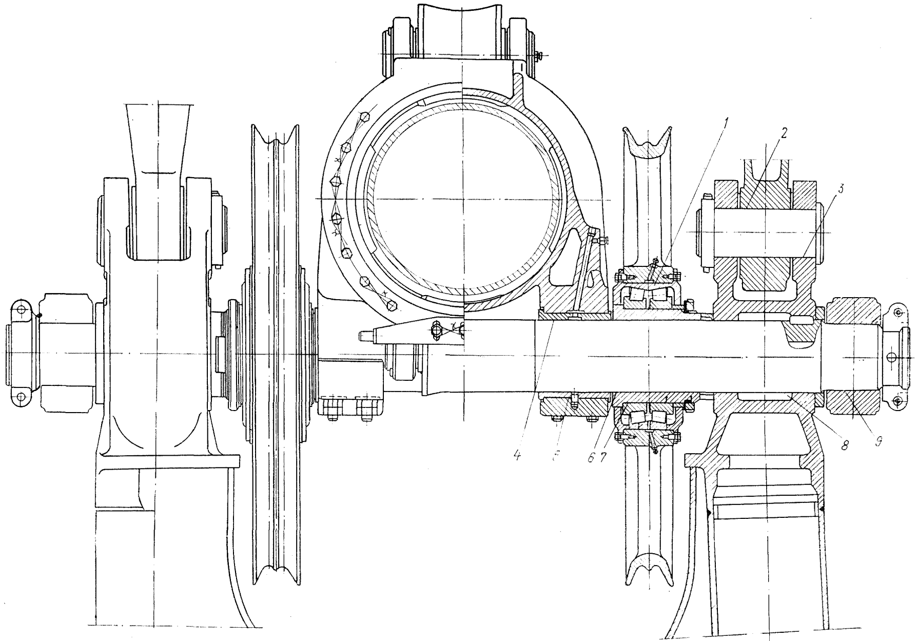
Рис. 6.4. Стрела и седловой подшипник
