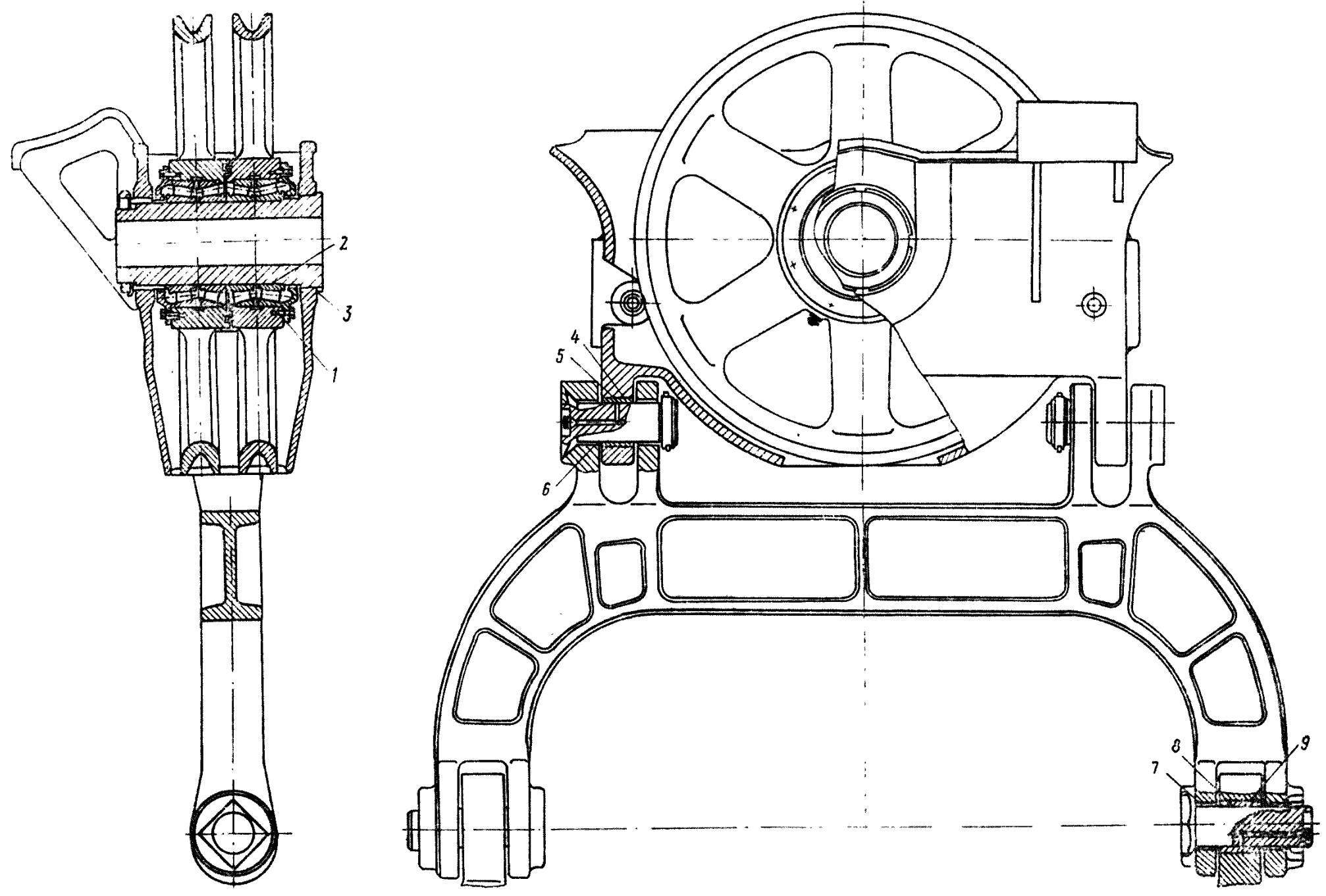
Рис. 6.2. Подвеска ковша
