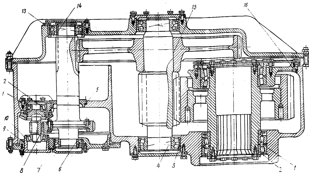
Рис. 6.16. Ходовой механизм
