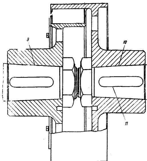
Рис. 6.12. Муфта моторная
