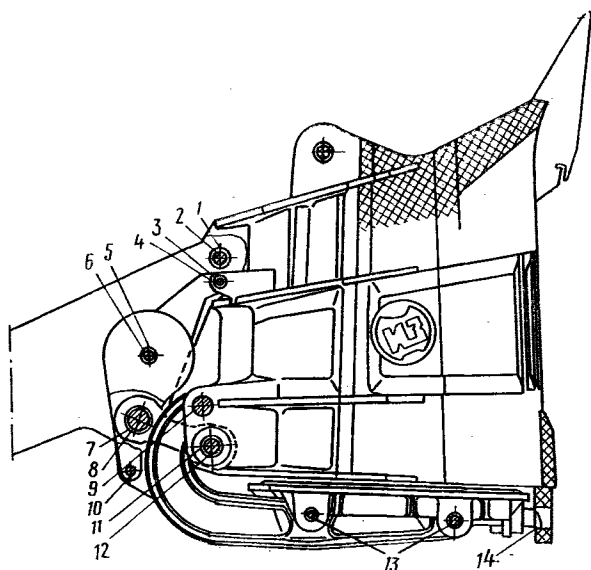
Рис. 6.1. Ковш
