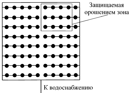
Рисунок Е.2 - Распределительная сеть с односторонней связью ветвей
