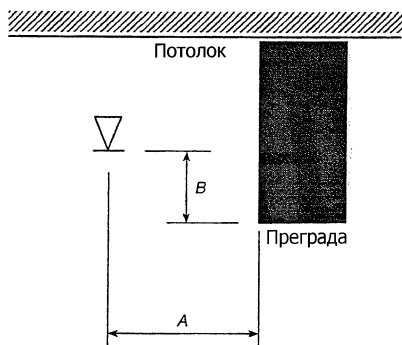
Рисунок 4.1- Расположение оросителя относительно его оси до преграды и от розетки до нижней поверхности преграды
