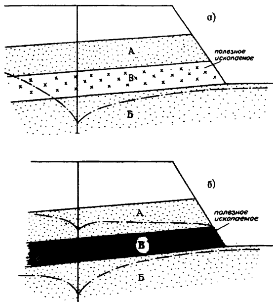
Рис. 19. Схемы дренажа рабочего борта водоупонизительными скважинами.
