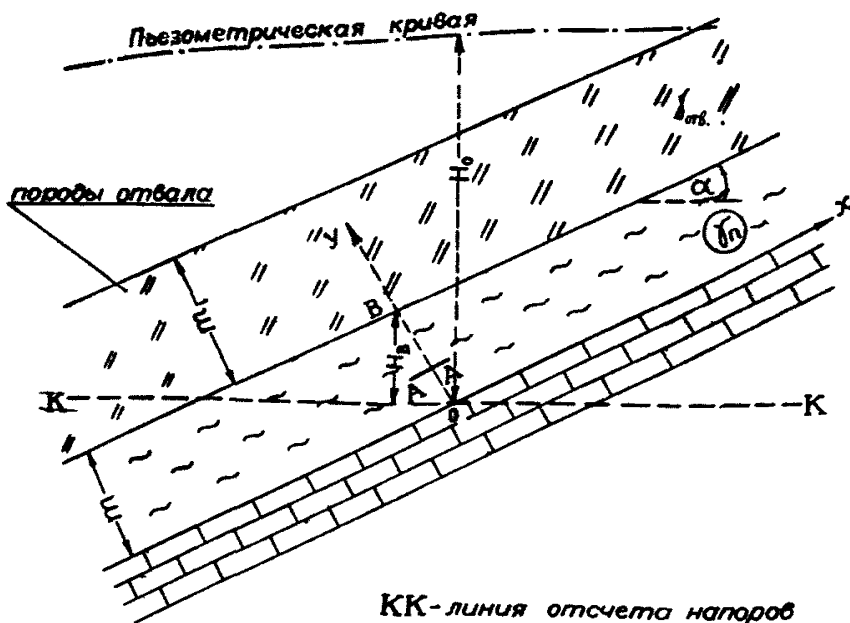
Рис. 1. Схема к определению "эффективных напряжений".
