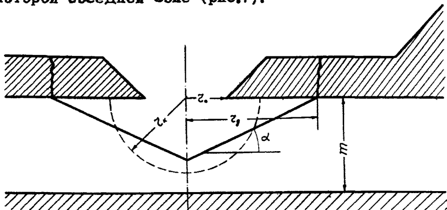
Рис. 7. Схема к расчету размеров деформированной зоны
