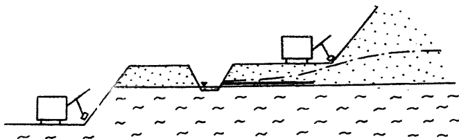
Рис. 17. Схема дренажа рабочего борта горизонтальными скважинами.
