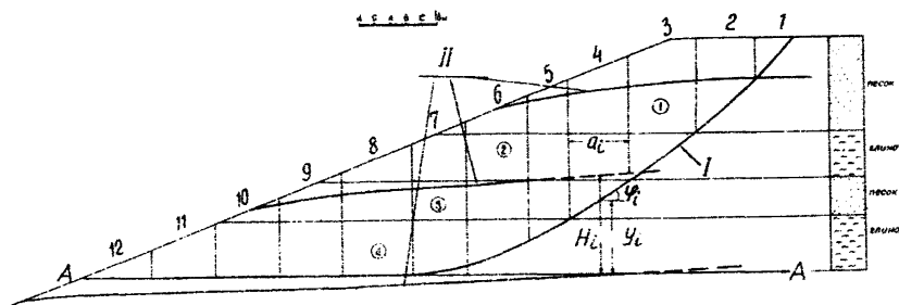
Рис.23. Схема к расчету устойчивости обводненного многослойного откоса
