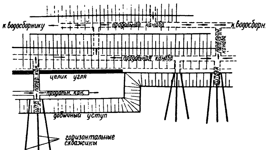
Рис. 21. Схема дренажа основания отвалов.
