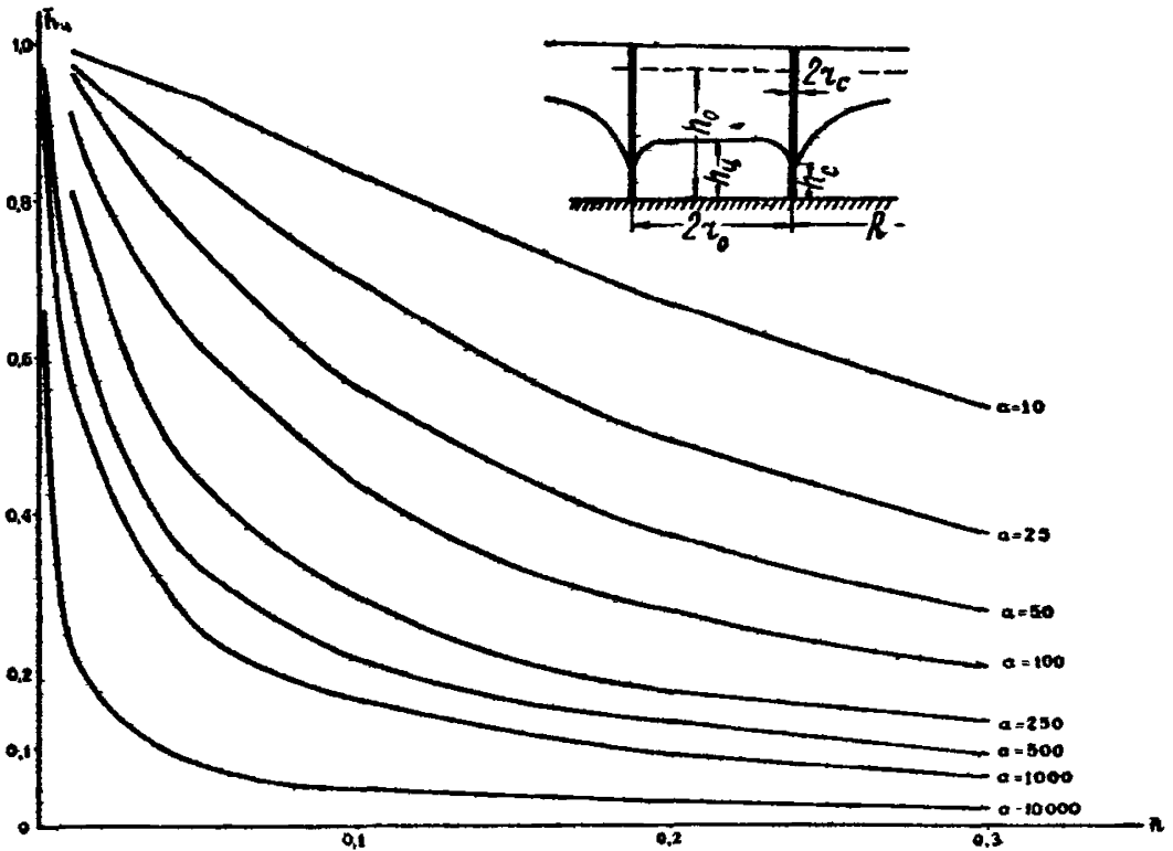
Рис. 15. График функции \bar{h}_u = f(\bar{n}) ; \bar{h}_u = \frac{h_u}{h_0} ; \bar{n} = \frac{\pi r_c^2}{r_0^2} ; a = \frac{r_0}{r_c} \ln \frac{R}{r_0} ; h_c^2 < h_0^2
