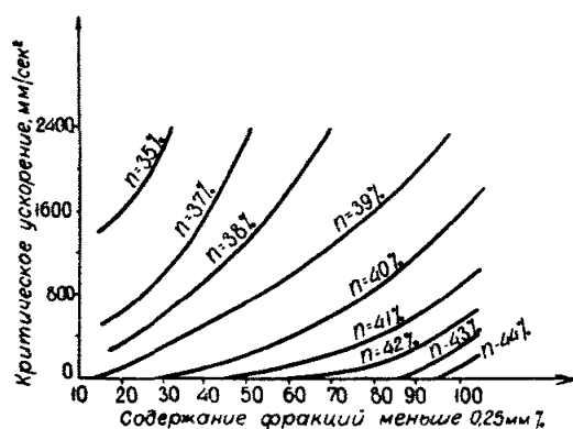
Рис. 8. Зависимость критического ускорения a_{кр} от механического состава и пористости песков ( n )
