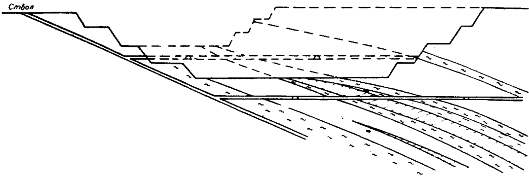
Рис. 20. Осушение карьера дренажными выработками, пройденными из наклонного ствола
