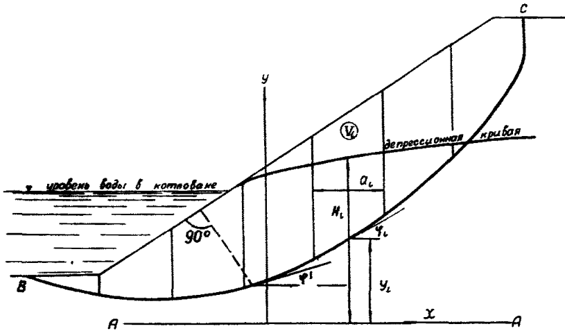
Рис. 2. Схема к расчету устойчивости обводненного откоса.
