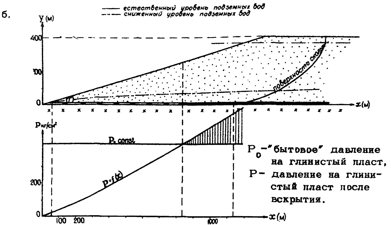
Рис. 4. Элюры распределения давлений на глинистый пласт:
