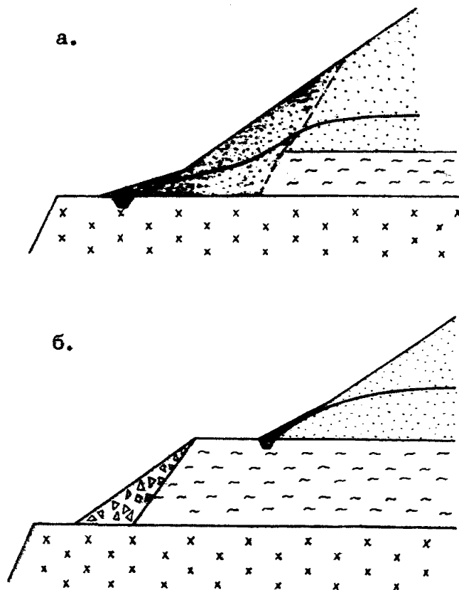
Рис. 13. Схемы пригрузки нерабочего уступа глинистых пород.
