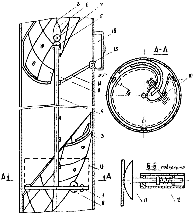
Рис. 11.5. Устройство для транспортирования грузов по однопутному следу
