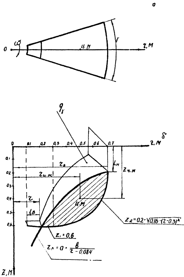
Рис. П.1. Угловой объем в проекции на горизонтальную плоскость (а) и схема определения геометрических и динамических параметров углового объема (б)
