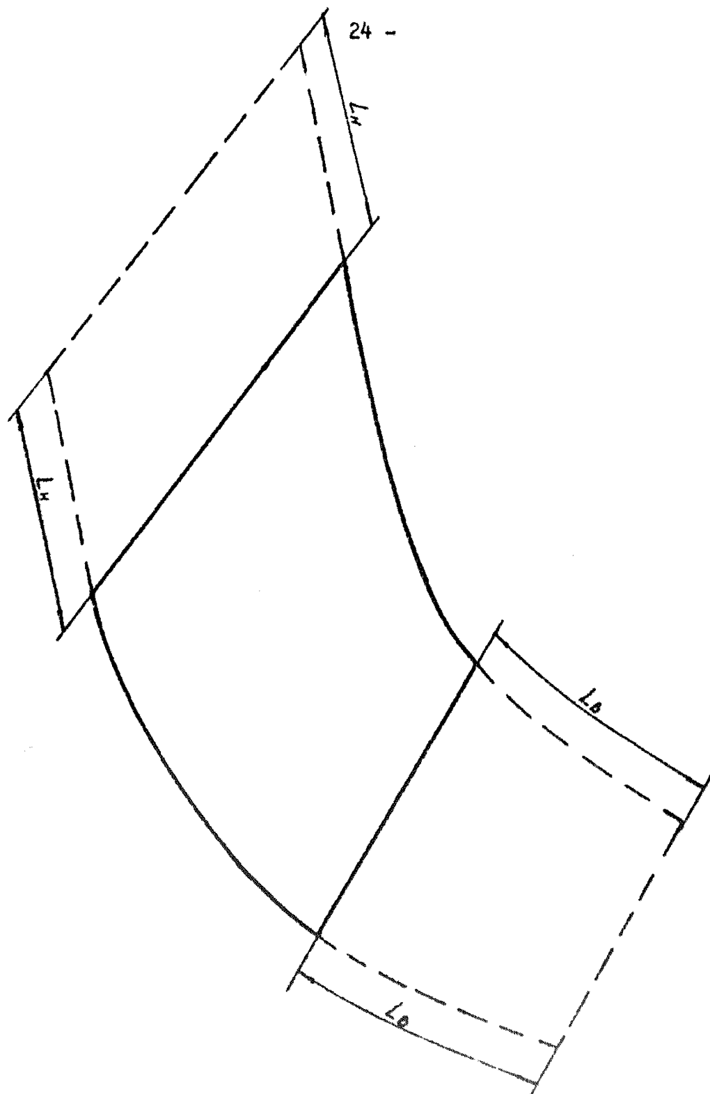
Рис. П.3. расположение вкладыша на развертке сектора спирали, защищающего его от износа
