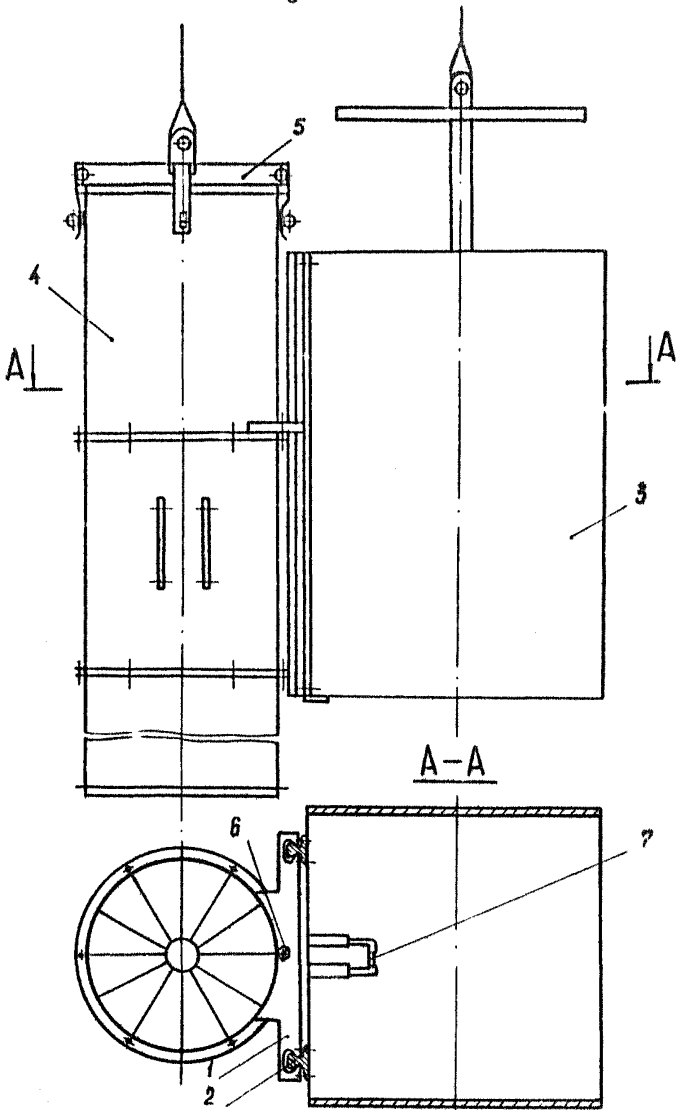
Рис. 3.2. Устройство фиксации
