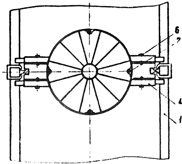
Рис. 3.1. Элементы крепления секций сноса
