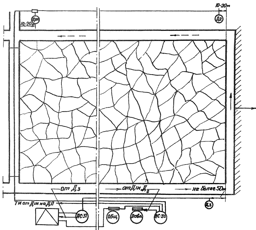
Рис 11. Схема размещения аппаратуры АГЗ при сплошной системе разработки (либа-штрек) на пластах пологого и наклонного падения, плоских по взвратным выбросам.
