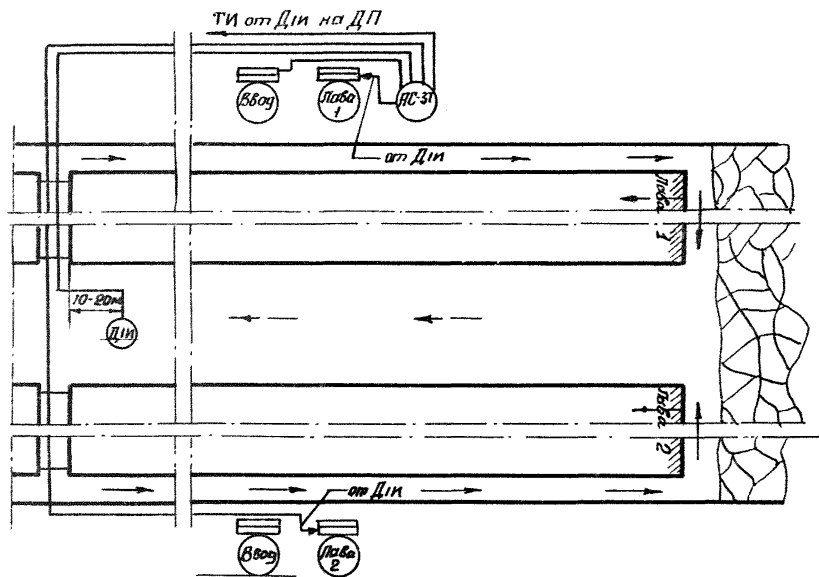
Рис 15. Схема размещения аппаратуры АГЗ при столбовой системе разработки (старенные лабры с общей исходящей струей).
