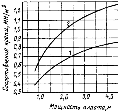
Рис. 1. Зависимости необходимого сопротивления механизированной крепи от мощности пласта и класса кровли: 1 - для кровли средней трудности управляемая (II класса); 2 - для трудноуправляемой кровли (III класса)
