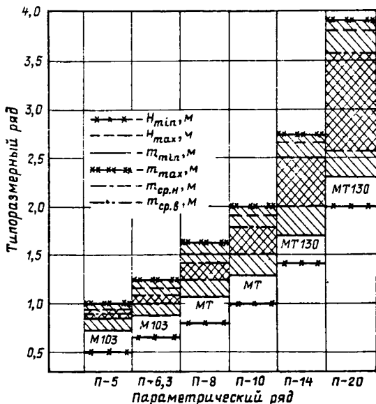
Рис. 3. Рациональная область применения механизированных крепей с предложенными параметрическим и типоразмерным рядами
