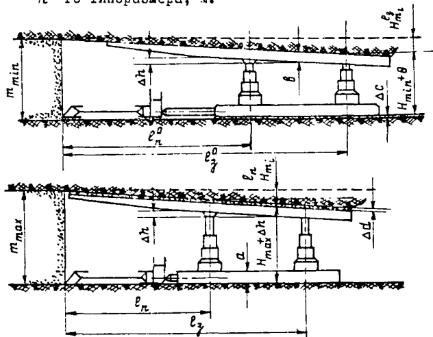
Рис. 2. Схема для расчета параметрического и типоразмерного рядов механизированных крепей
