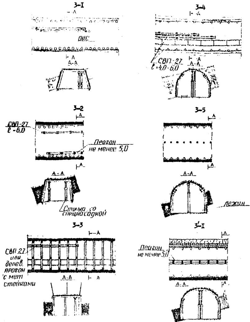
Рис. 9.8. Типовые схемы установки усиливающей крепи в подготовительных выработках впереди очистного забоя
