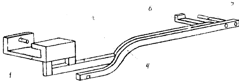
Рис. П.5.3. Приспособление ПНВ-4 для навески верхняков В20Б: 1- захват; 2- фиксирующее устройство; 3- кронштейн; 4- рычаг; 5- валик рычага; 6- площадка кронштейна
