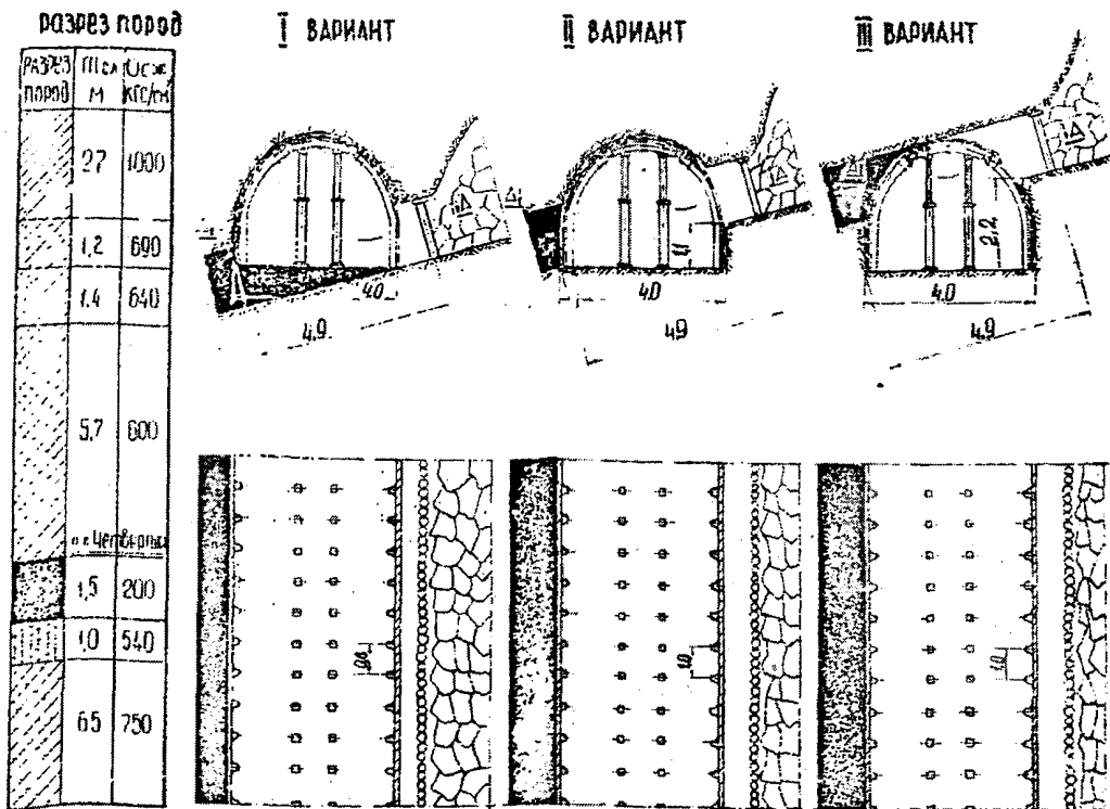
Рис. П.9.4. Строение и прочность боковых пород пласта Четвертого, варианты расположения конвейерного штрава относительно кровли и почвы пласта и средства поддержания выработки позади лавы
