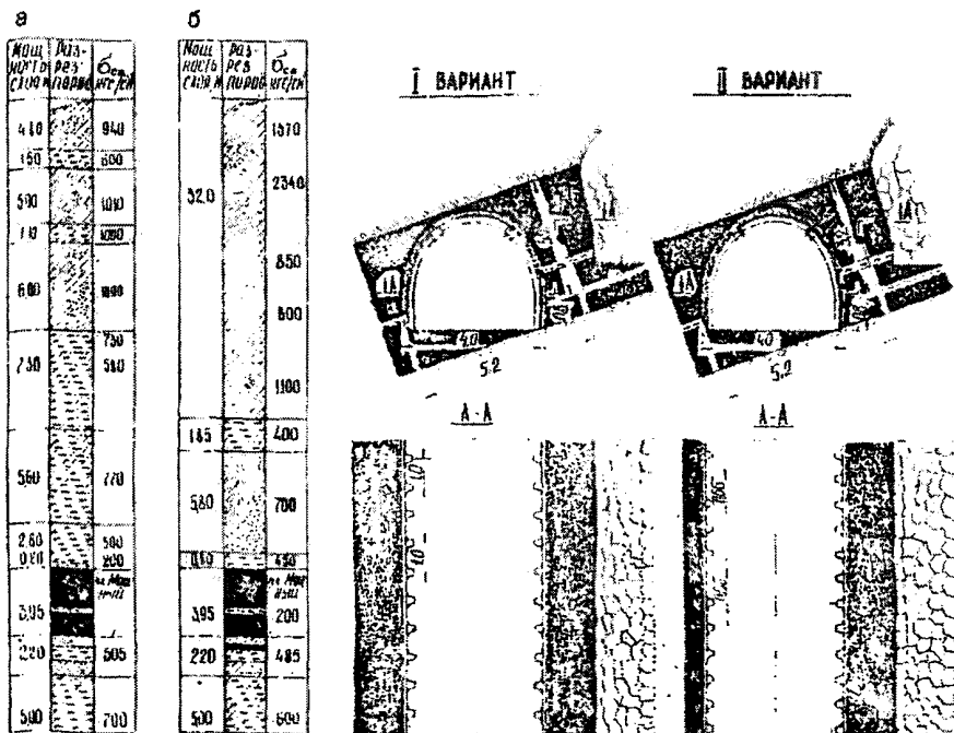
Рис. П.9.5. Необходимая плотность установки металлической арочной крепи в вентиляционном штреке пласта Мошного при среднеобрушаемой (а, I вариант) и труднообрушаемой (б, II вариант) кровлях
