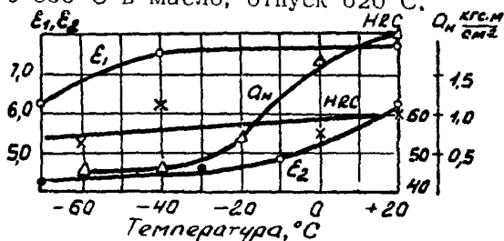
Рис. 22. Сталь 60С2А, закалка с 870°С в масло, отпуск 200°С.
