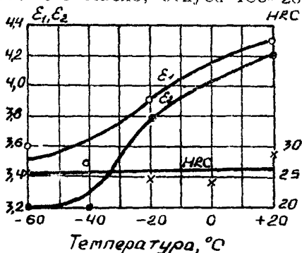
Рис. 21. Сталь 20ХН4ФА, закалка с 850°С в масло, отпуск 620°С.
