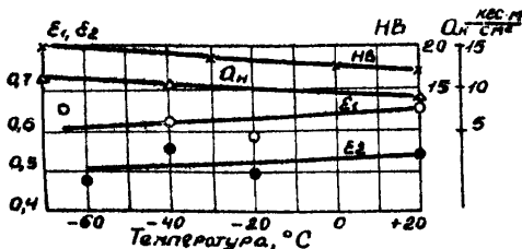
Рис. 3. Алюминий, отжиг 380^{\circ}\text{C} .
