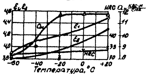
Рис. 17. Сталь 40XН 1 , закалка с 820°С в масло, отпуск 470°С.
