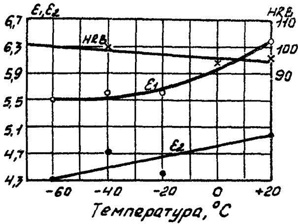
Рис. 28. Сталь 13X2БЛ, отжиг 820°С.
