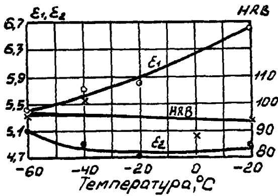
Рис. 28. Сталь 13X2БЛ, отжиг 820°С.
