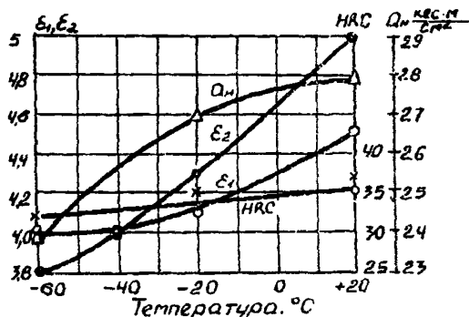
Рис. 20. Сталь 12Х2Н4А, закалка с 780–800°С в масло, отпуск 180–200°С.
