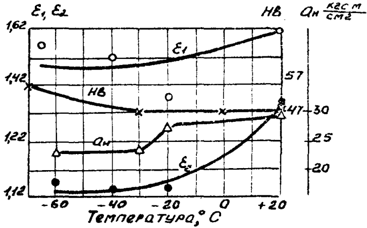
Рис. 5. Медь, отжиг 650°С.
