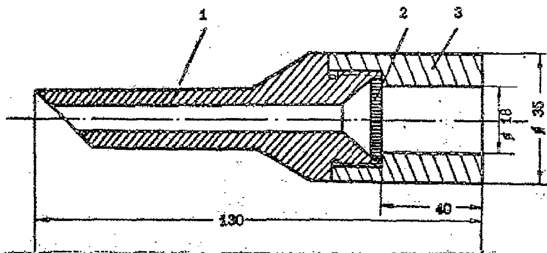
Рис. 13. Разъемная воронка: 1 - корпус; 2 - фильтр; 3 - стакан
