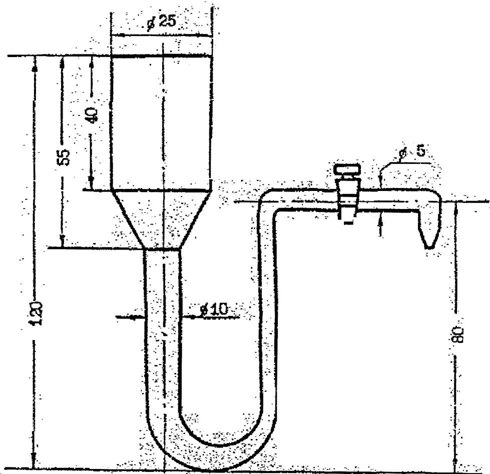
Рис. 12. Колонка для определения 239 Pu
