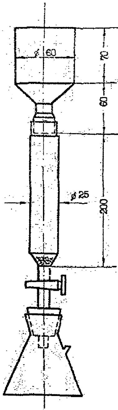
Рис. 9. Колонка для определения ^{131}\text{I}
