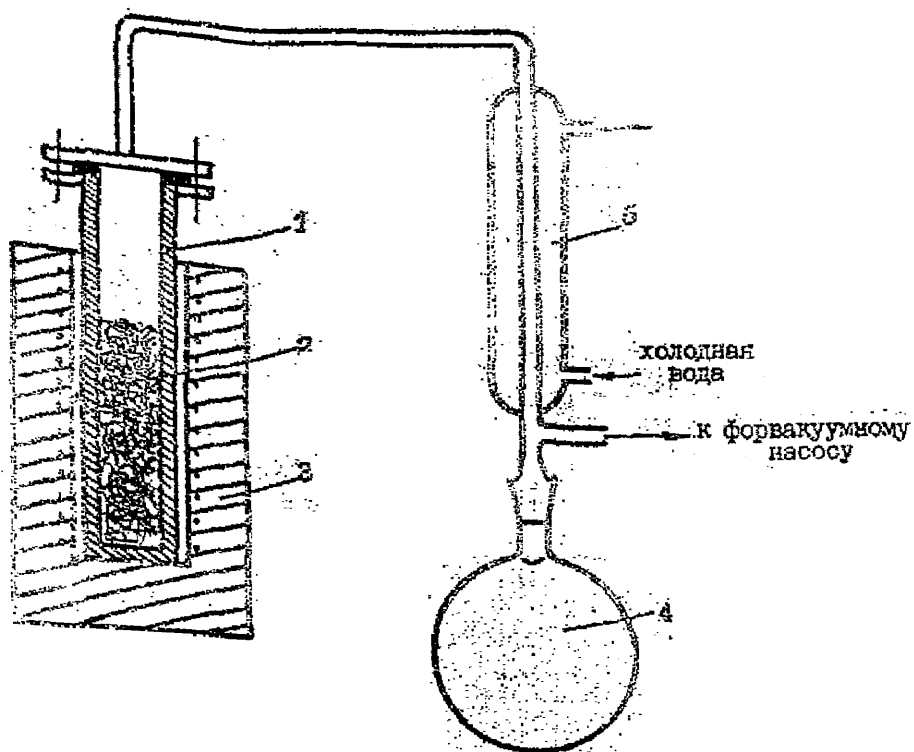
Рис. 5. Аппарат для обугливания исследуемого материала. 1 - реактор; 2 - исследуемый образец; 3 - шахтная печь; 4 - колба для сбора летучих продуктов; 5 - холодильник
