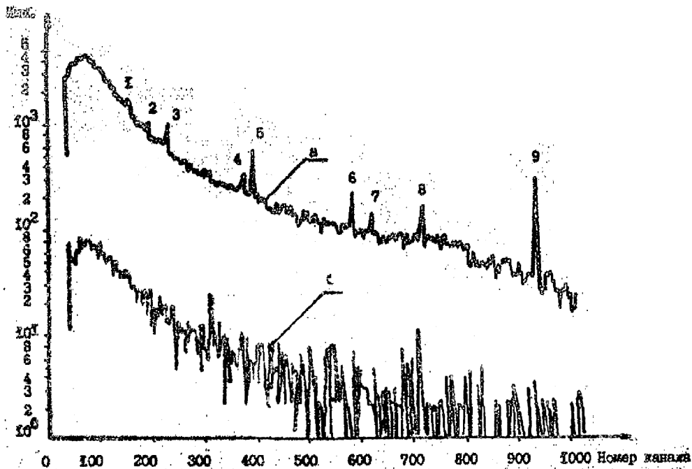
Рис. 19. Аппаратурные спектры естественного фона:
