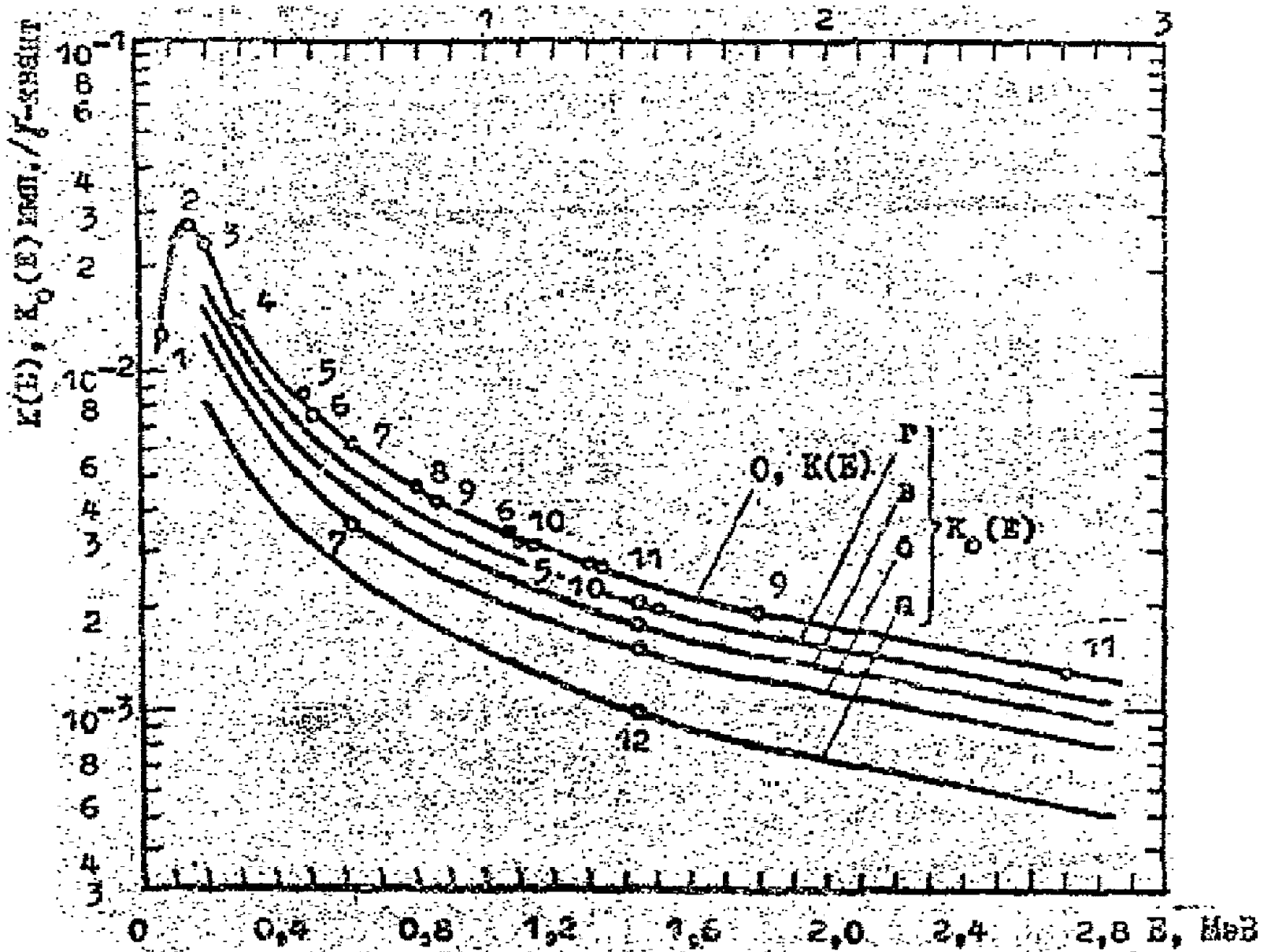
Рис. 31. Эффективность регистрации различных \gamma -квантов для проб различных объемов при отсутствии самопоглощения излучения:
