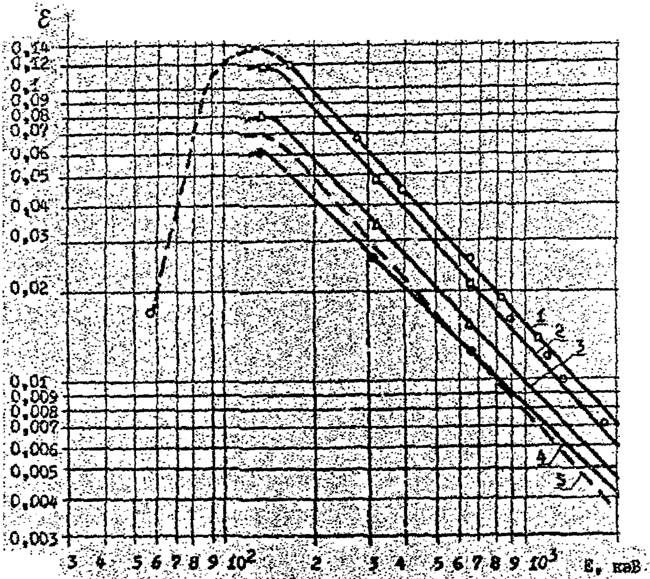
Рис. 26. Зависимости абсолютной эффективности регистрации от энергии \gamma -квантов для препаратов различных объемов: 1 - 0,01 мл; 2 - 0,5 мл; 3 - 4 мл; 4 - 14 мл; 5 - 14 мл
