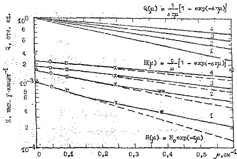
Рис. 29. Калибровочные кривые N(\mu) и Q(\mu) для проб различных объемов:
