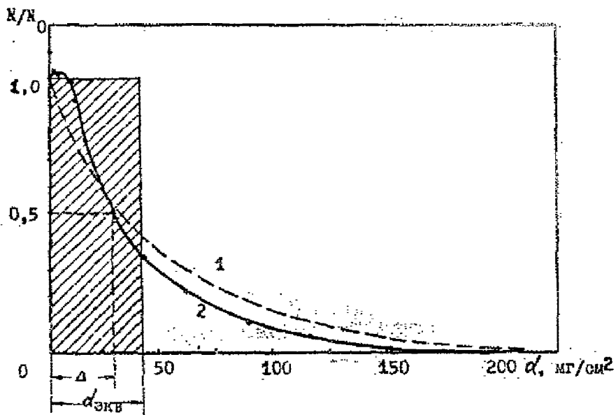
Рис. 15. Определение эквивалентной толщины слоя ослабления материала по кривой поглощения: 1 — экспонента; 2 — кривая поглощения
