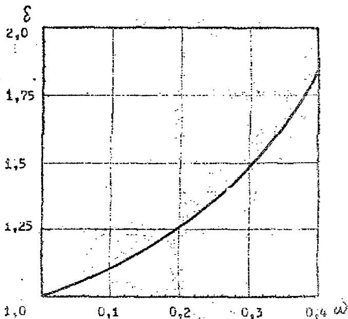
Рис. 16. График зависимости поправки на "косые лучи" ( \delta ) от величины телесного угла ( \omega )
