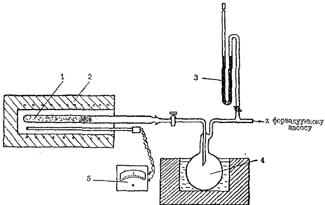
Рис. 4. Схема прибора для активации катализатора:
