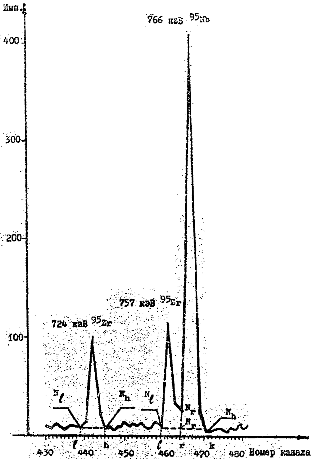
Рис. 25. Участок аппаратурного спектра, обусловленного \gamma -излучением ^{95}\text{Zr} + ^{95}\text{Nb} .
