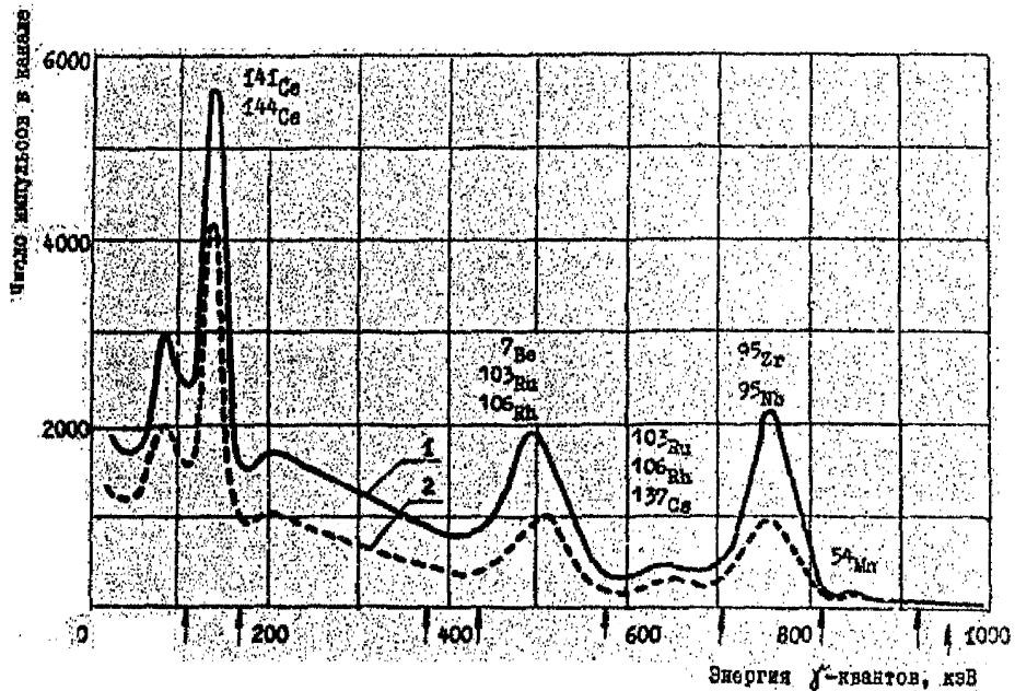
Рис. 32. \gamma -Спектр пробы аэрозолей, содержащей продукты деления возрастом около 6 месяцев:
