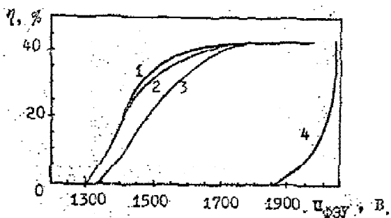
Рис. 17. Счетная и шумовая характеристика прибора SAS-P-2:
