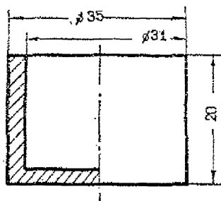
Рис. 10. Счетная кювета.
