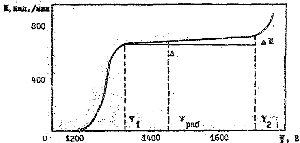
Рис. 14. Вид счетной характеристики газоразрядного счетчика
