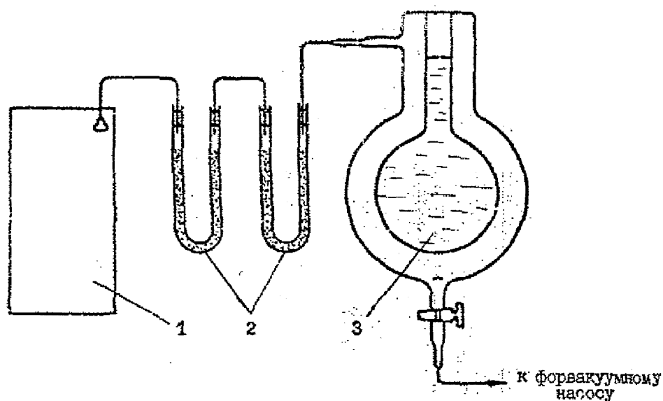
Рис. 7. Схема очистки ацетилена:
