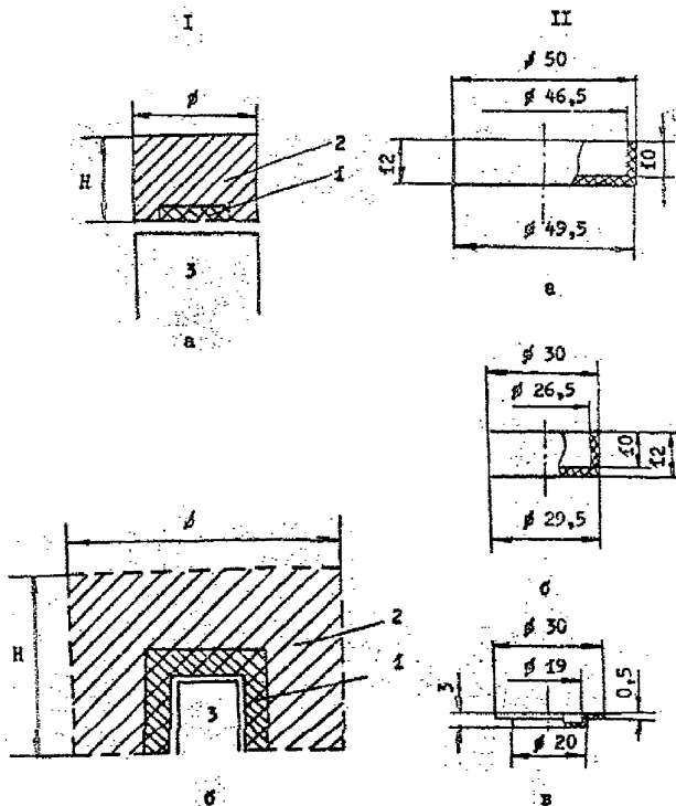
Рис. 21. Геометрия объемных проб:
