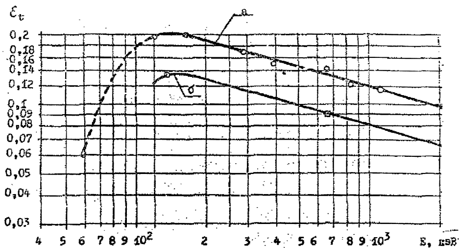
Рис. 27. Зависимости полной эффективности регистрации от энергии \gamma -квантов для препаратов различных объемов:
