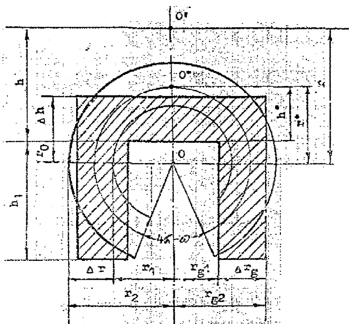
Рис. 28. Геометрия стаканобразной и эквивалентной ей сферической формы проба:
