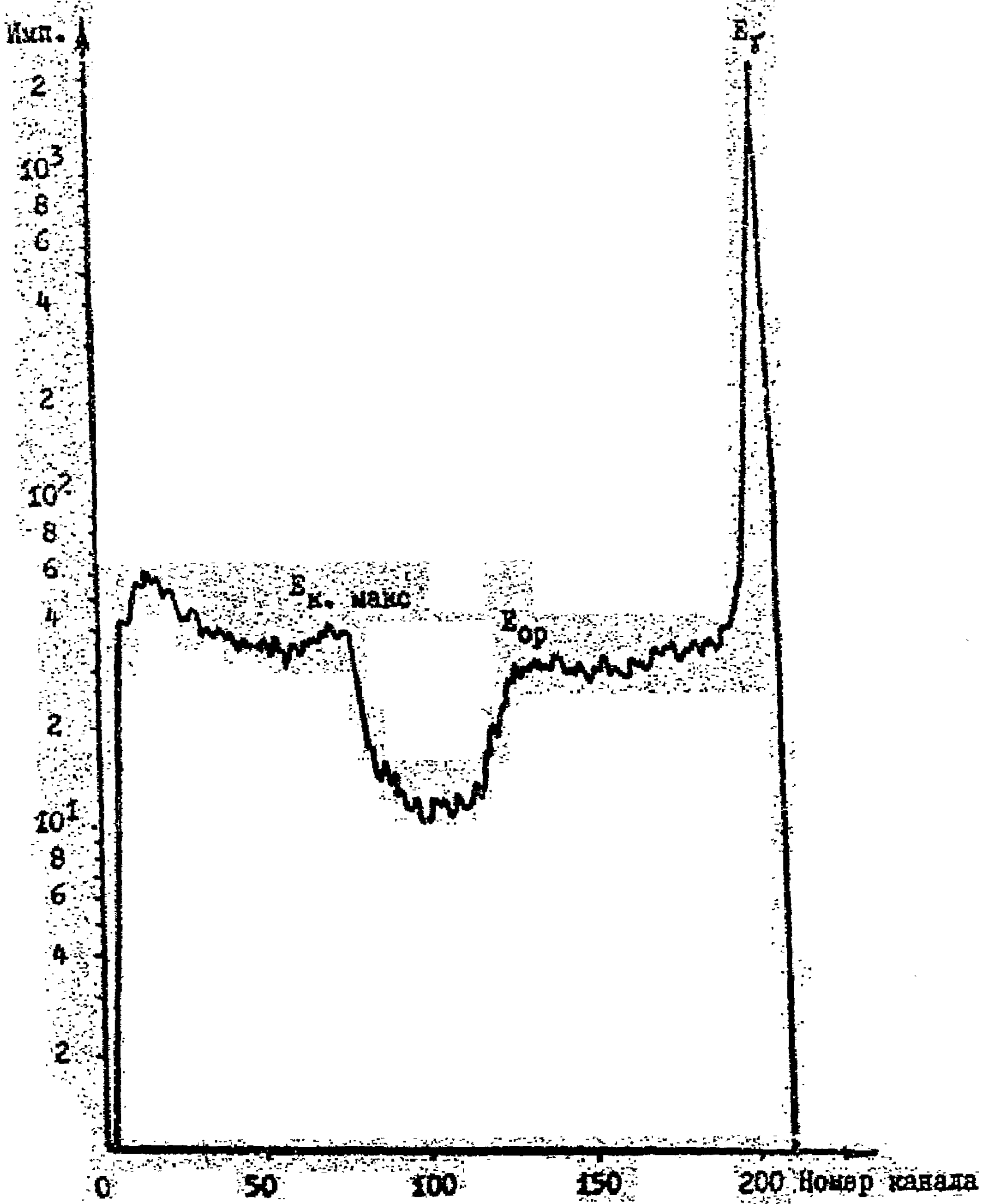
Рис. 23. Аппаратурный спектр \gamma -излучения ^{139}\text{Ce} .
