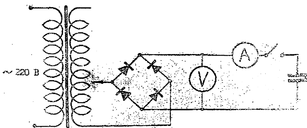
Электрическая схема установки для электролиза
