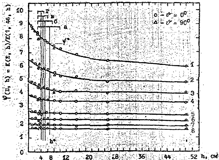
Рис. 30. Зависимость относительной эффективности регистрации J -квантов точечного источника от расстояния источника
