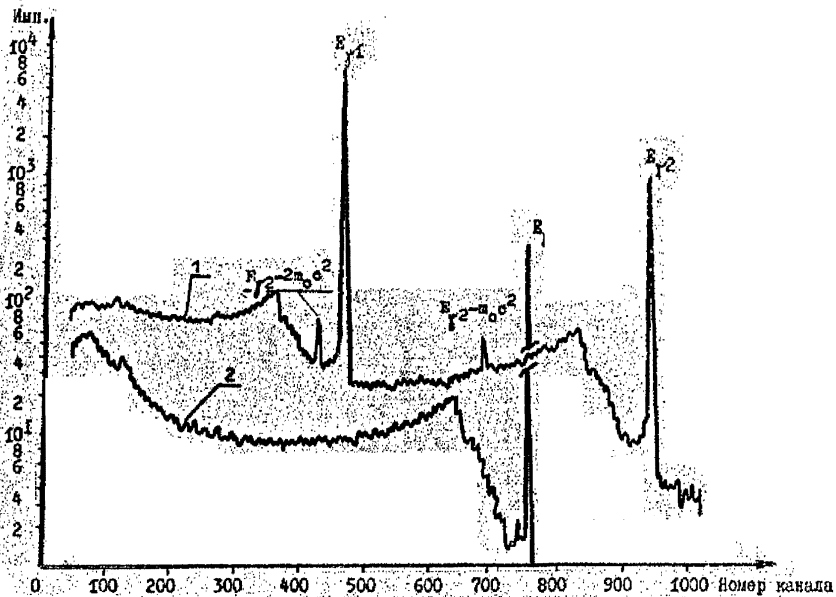
Рис. 24. Аппаратурные спектры \gamma -излучения ^{88}\text{Sr} (1) и ^{40}\text{K} (2)
