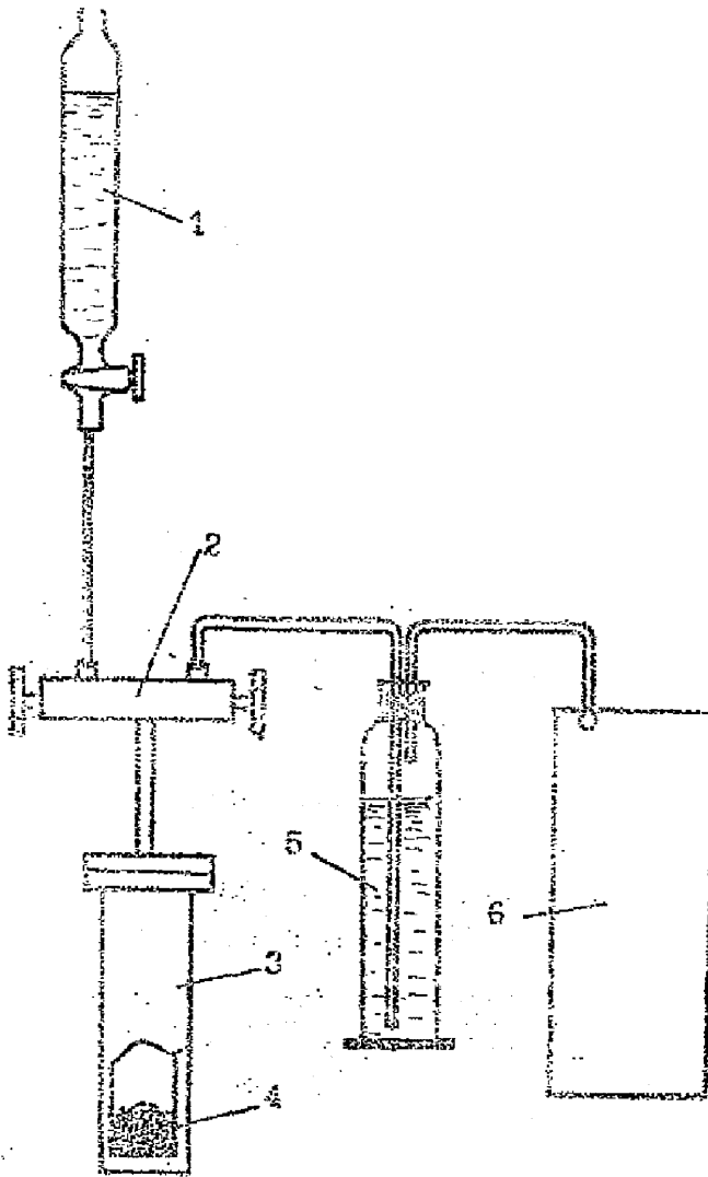
Рис. 6. Схема установки для разложения кар-
