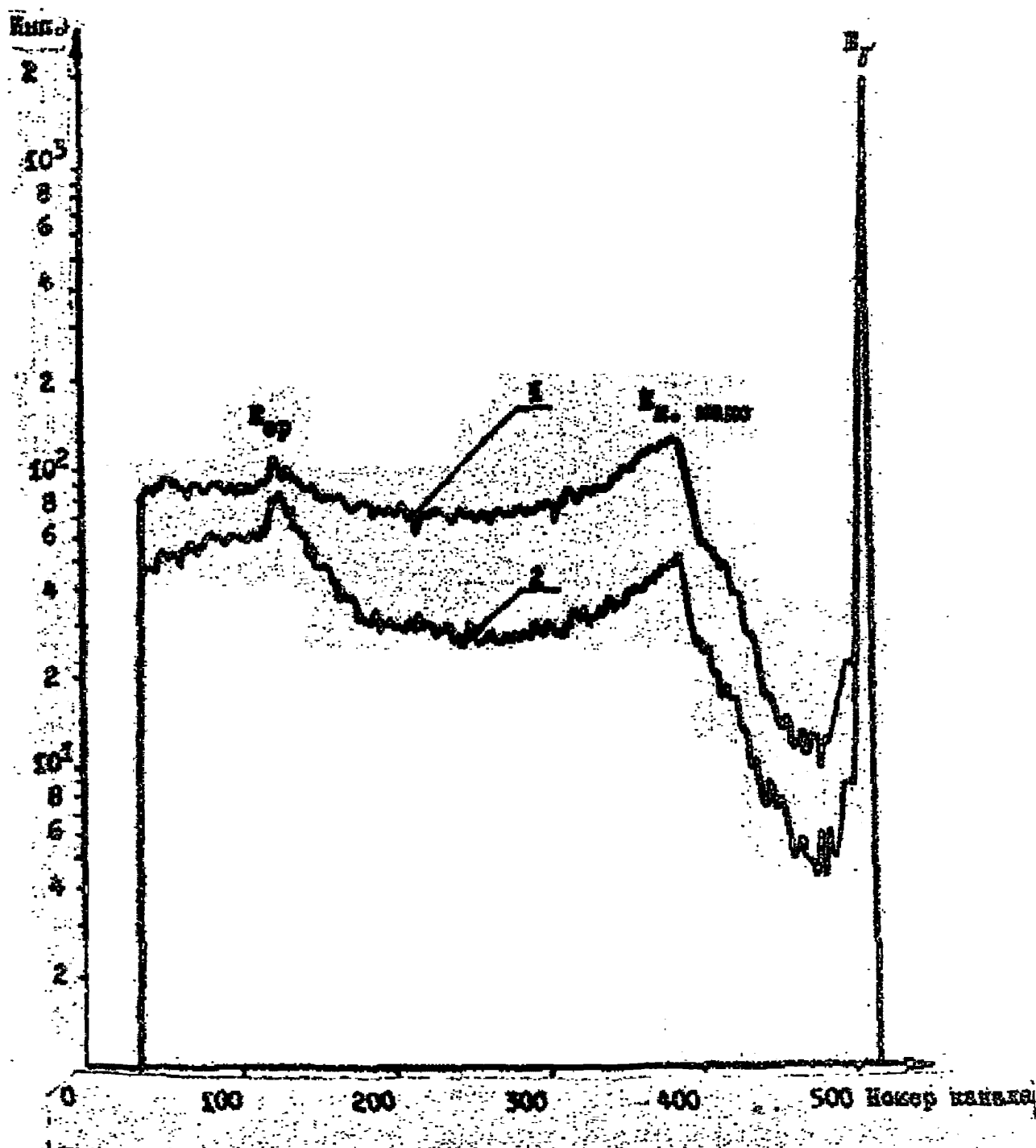
Рис. 22. Аппаратурные спектры \gamma -излучения ^{59}\text{Fe}
