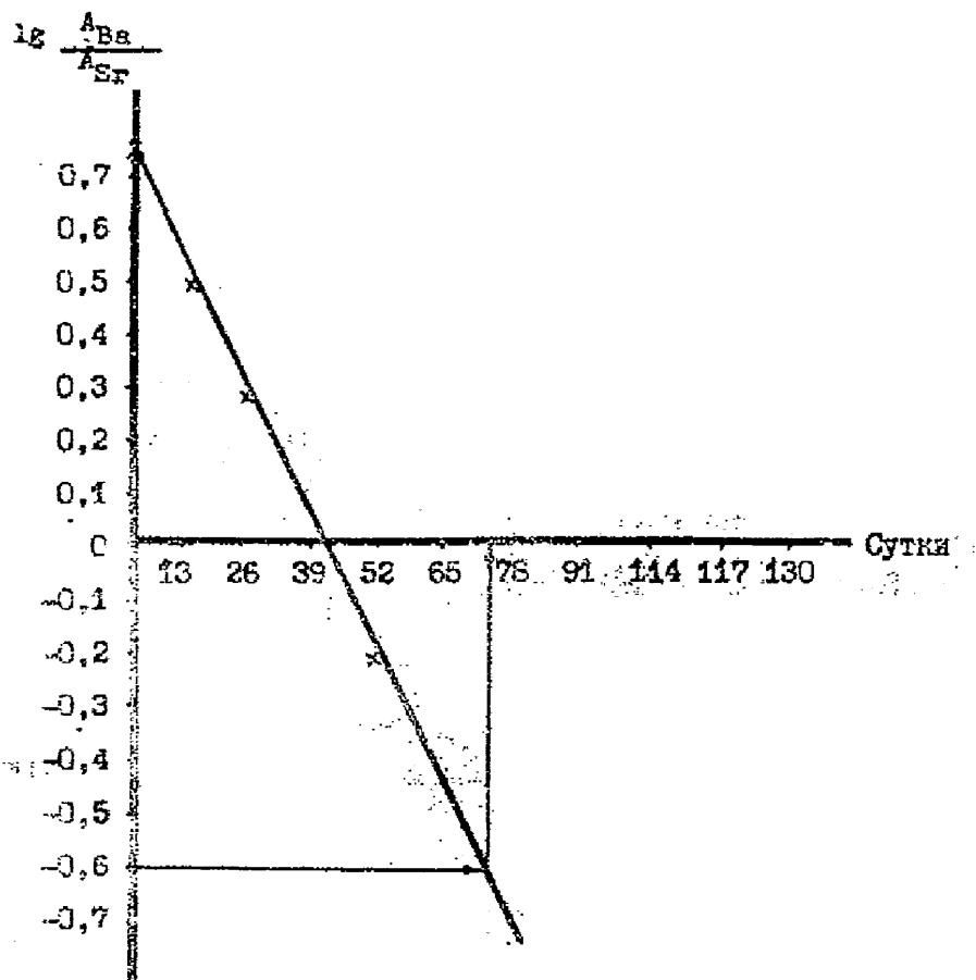
Рис. 2. Изменение отношения активностей ^{140}\text{Ba} и ^{89}\text{Sr} со временем.
