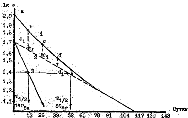
Рис. 1. Кривая распада и ее графический анализ:
