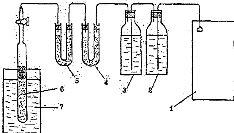
Рис. 8. Схема синтеза бензола:
