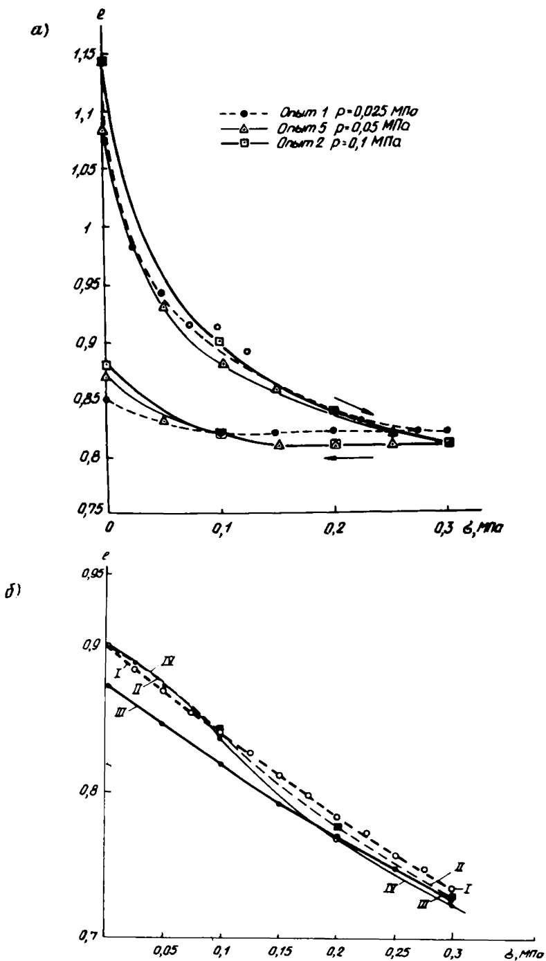
Рис. 8. Компрессионные кривые а — пасты каолиновой глины ( w = w_{s\omega} ); б — суглинок пылеватый с ненарушенной структурой
