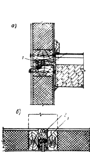
Рис. 4. Примеры конструктивных решений стыков панелей для жилых зданий
