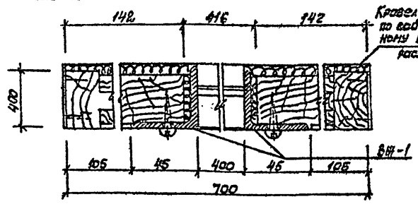
Сечение II-II
