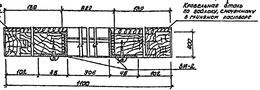
Сечение II-II
