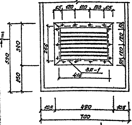
Сечение II-II
