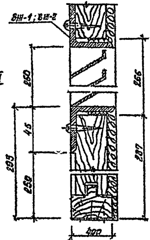
Сечение I-I
