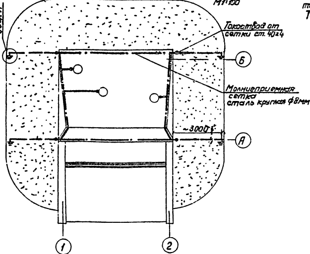
План молниеприемной сетки и заземлителя М1:100
