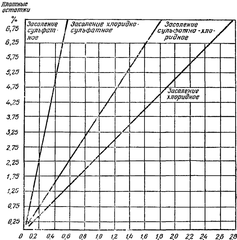
Рис. Определение типа засоления по соотношению плотного осадка и хлора (по Б. А. Калачеву). На оси абсцисс указано содержание хлора в %.
