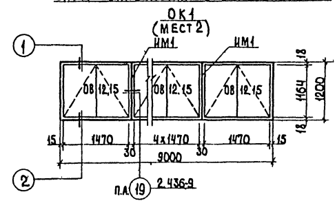
СХЕМА ЗАПОЛНЕНИЯ ОКОННОГО ПРОЕМА
