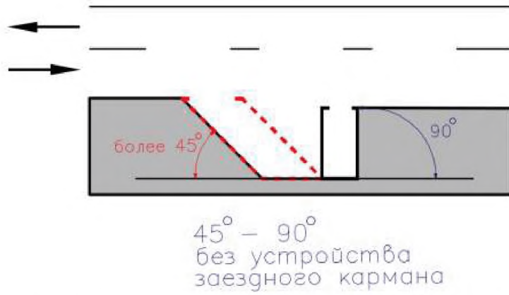
Рисунок 20 - Рекомендации по размещению парковки в интервале от 46° до 90° в заездном кармане
