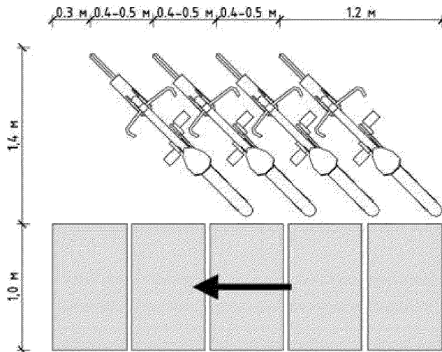
Рисунок 2.2. Диагональное расположение велосипедов
