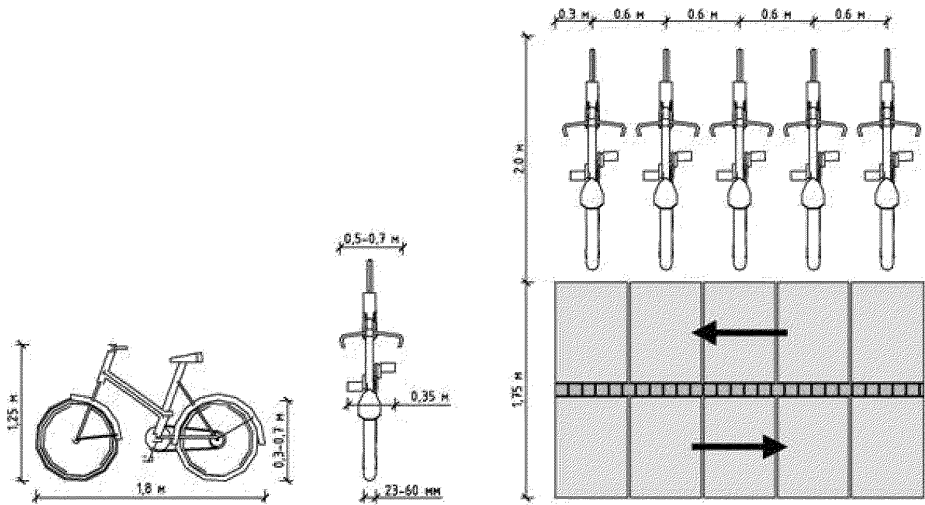
Рисунок 2.1. Рекомендуемые размеры велопарковки
