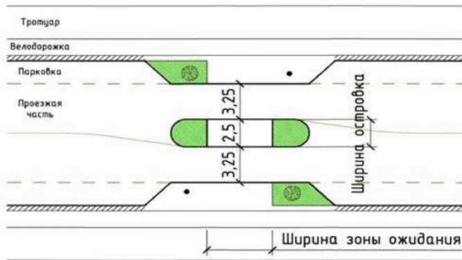
Рисунок 4.2. Пример устройства центрального островка на проезжей части
