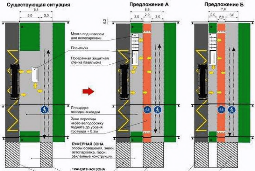
Рисунок 4.11. Рекомендации по планировочным решениям остановочного пункта
