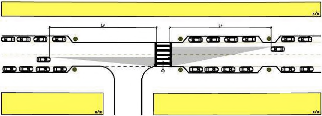
б) Рисунок 3.3. Поле видимости: а) - для обладающих преимущественным правом проезда водителей автомобилей и велосипедистов; б) - зона видимости в зоне пешеходного перехода и при пересечении проезжей части велосипедистами вместе с пешеходами
