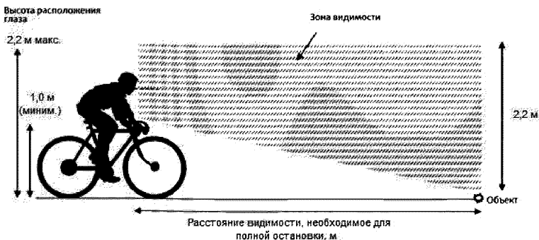
Рисунок 3.5. Зона вертикальной видимости для велосипедистов
