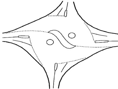
Рисунок 5.2 - Пересечение канализованного типа со сложной планировкой (Вариант №2)
