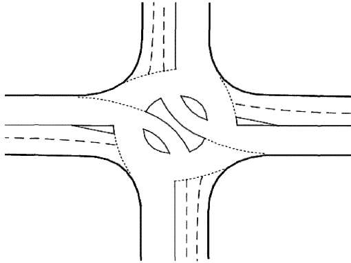
Рисунок 5.1 - Пересечение канализованного типа со сложной планировкой (Вариант №1)
