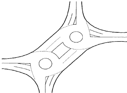
Рисунок 5.3 - Пересечение канализованного типа со сложной планировкой (Вариант №3)
