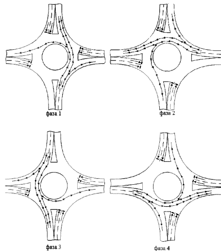
Рисунок 2.17 - Метод организации светофорного регулирования «Зелёная турбина»
