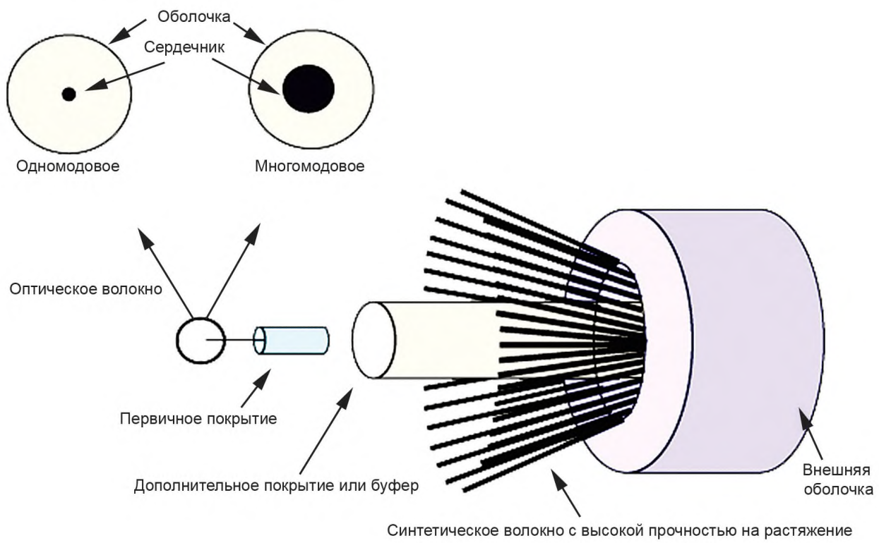
Рисунок D.2 — Типовая конструкция одноволоконного оптического кабеля
