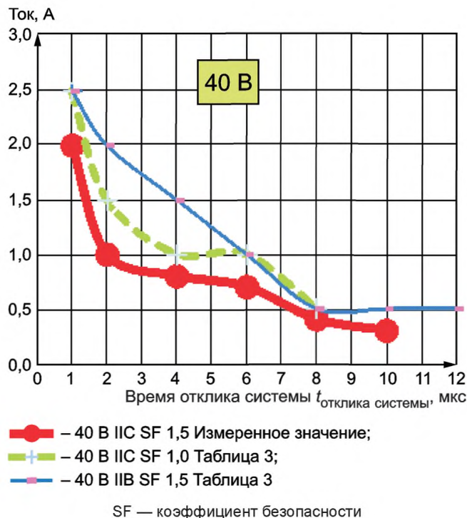
Рисунок В.10 — Значения воспламенения Power-і для класса напряжения 40 В (40 В постоянного тока)
