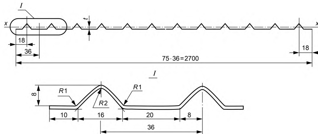
Рисунок 2 — Профили типа А высотой 8 мм
