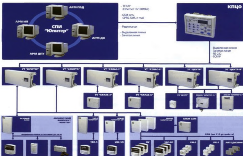
Структурная схема СПИ «Юпитер»
