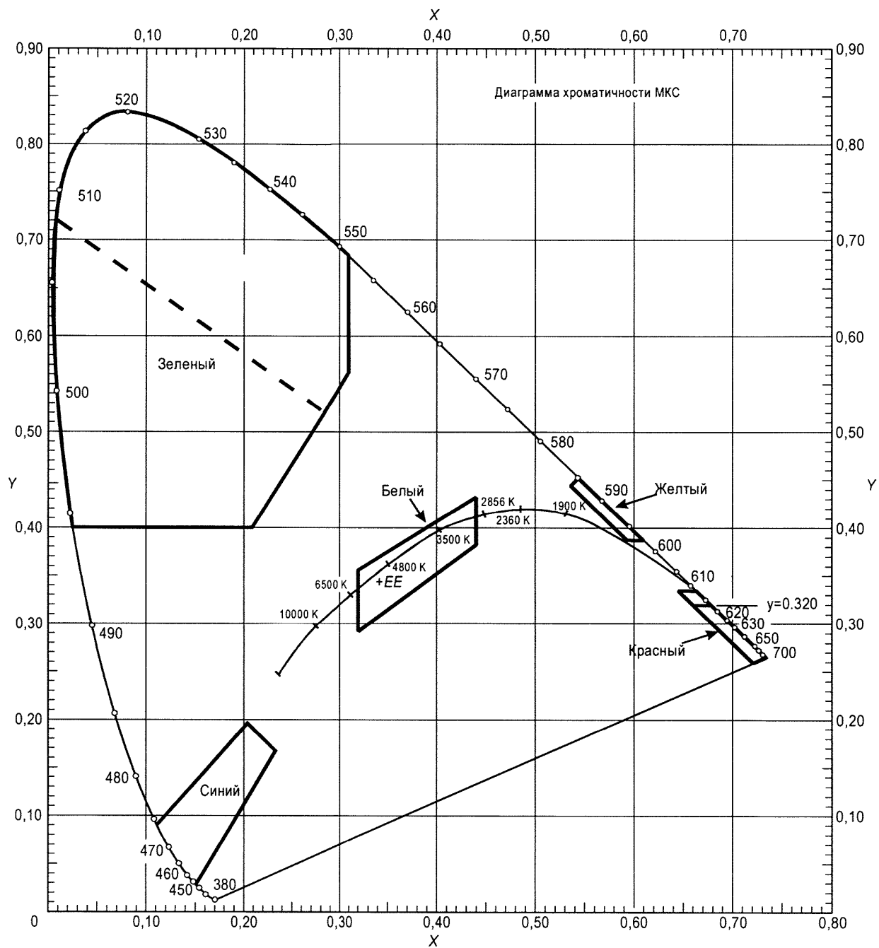
Рис. А1-1б. Цвета аэронавигационных наземных огней (твердотельные источники света)
