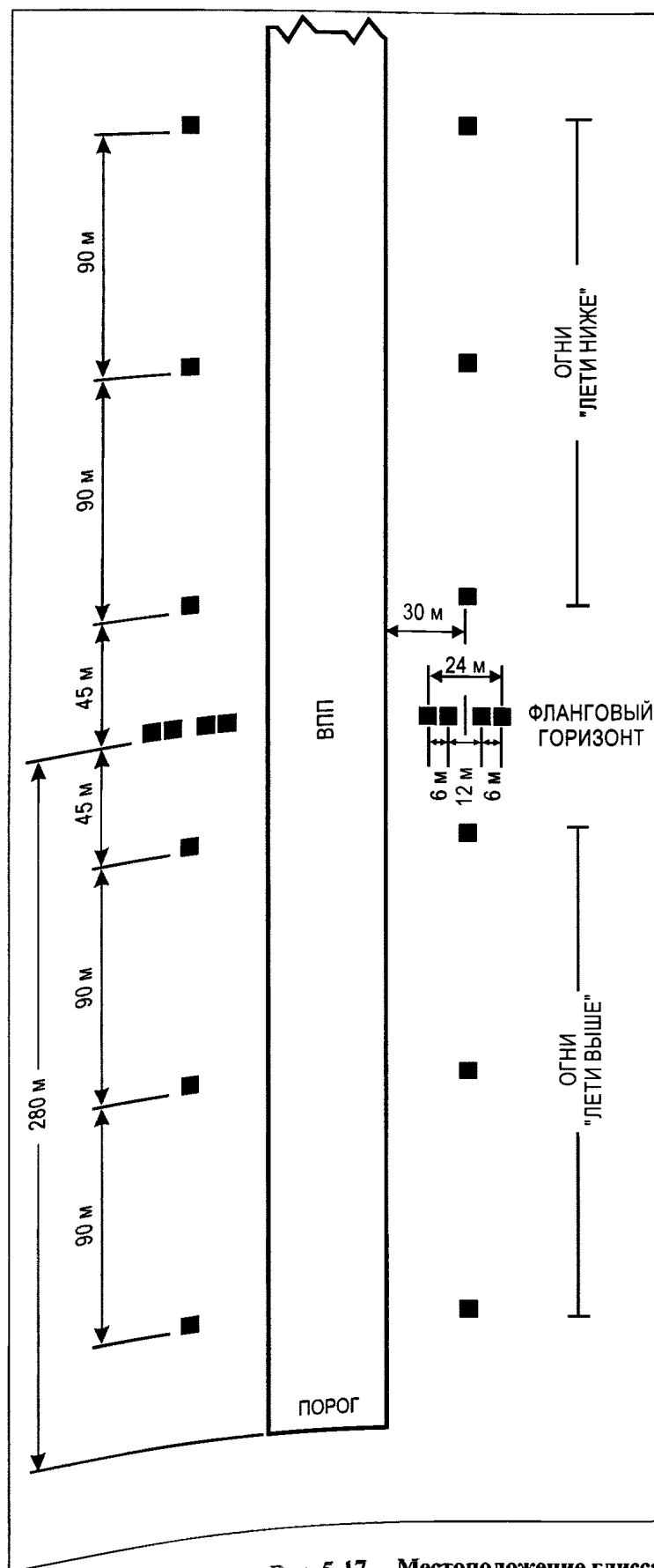
Рис. 5-17. Местоположение глиссадных огней системы T-VASIS
