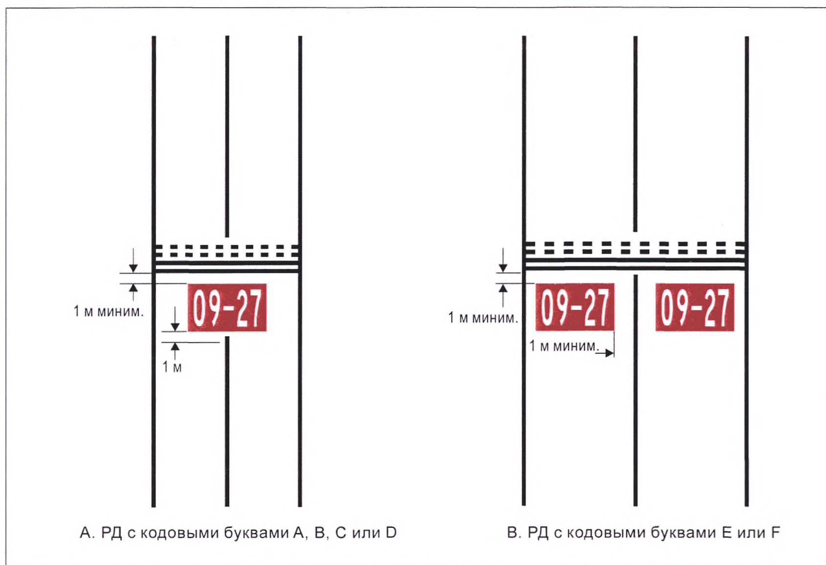
Рис. 5-10. Маркировка, содержащая обязательные для исполнения инструкции
