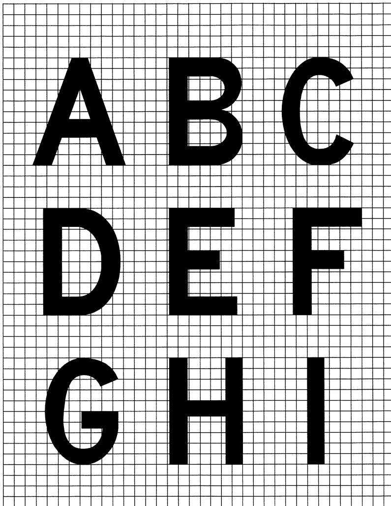
Рис. А4-2. Форма знаков
