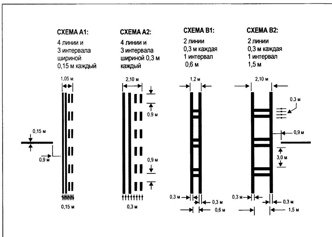
Рис. 5-8. Маркировка места ожидания у ВПП
