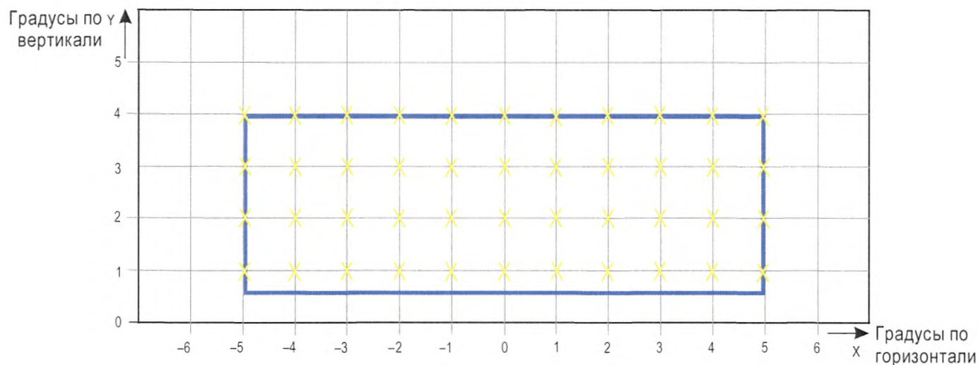
Рис. A2-21. Точки координатной сетки, предназначенные для вычисления средней силы света осевых огней РД и огней линии "стоп"
