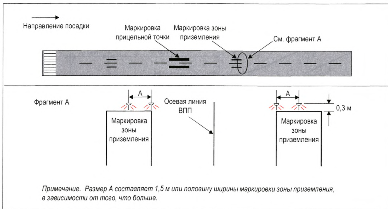
Рис. 5-24. Простые огни зоны приземления
