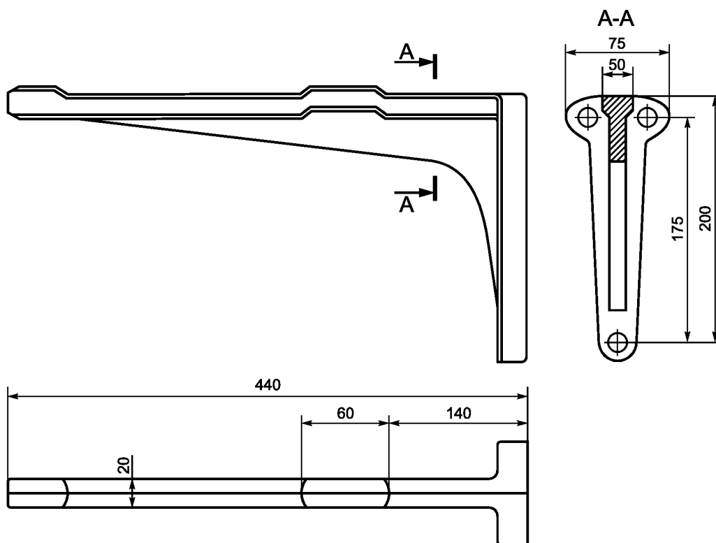
Рисунок 3 — Кронштейн чугунный для мойки, большой
