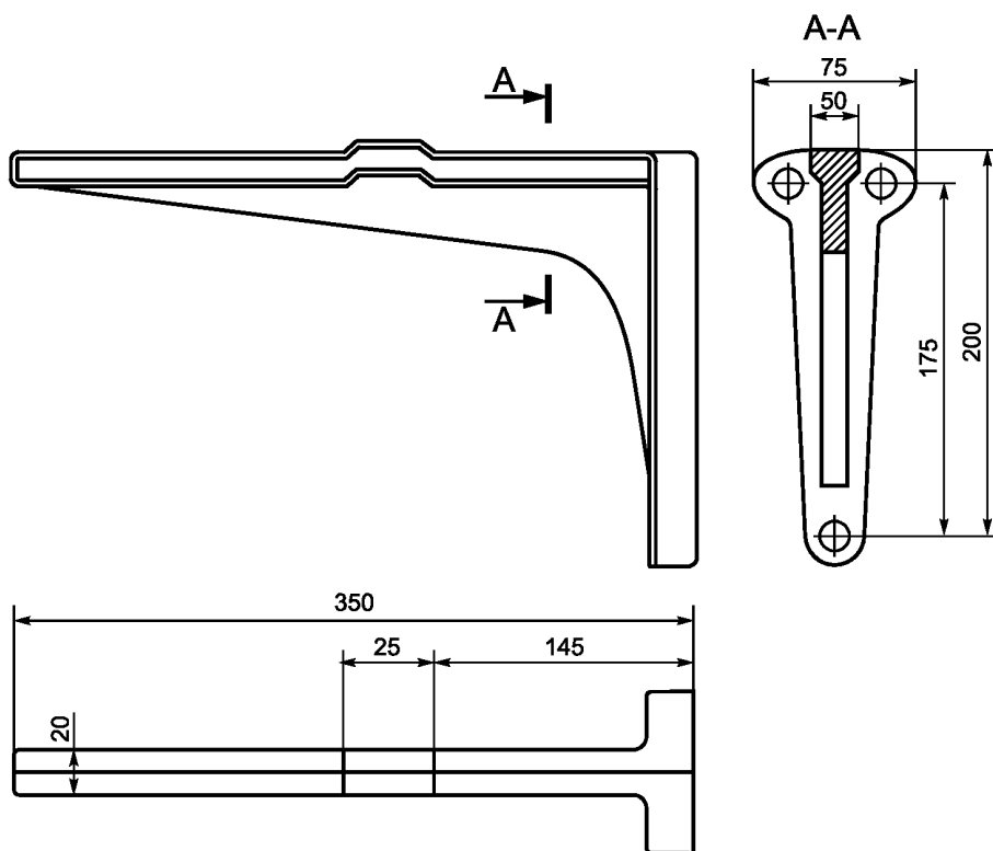
Рисунок 4 — Кронштейн чугунный для мойки, малый
