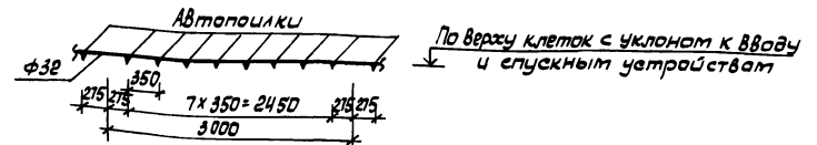
Фрагмент схемы системы Б31
