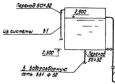
Схема установки водонапорного бака
