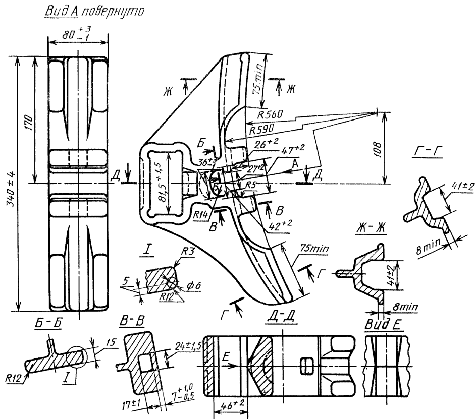
Условное обозначение неповоротного башмака Башмак неповоротный ГОСТ 3269—78 (ИУС № 11 1989 г.)
