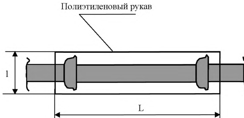
Рисунок А.16 – Полиэтиленовый рукав
