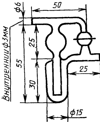
Склянка Дрекслея с краном
