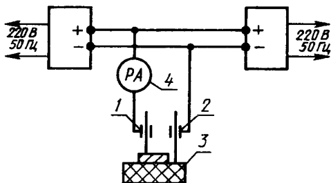
1, 2 — щипцовый зажим; 3 — платиновые сетчатые электроды (комплект); 4 — амперметр
