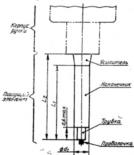
Рисунок 1 — Наконечник трубчатый
