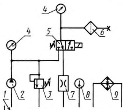
Схема стенда для ресурсных испытаний фильтра
