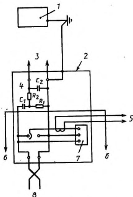
Рекомендуемая схема генератора импульсного испытательного напряжения
